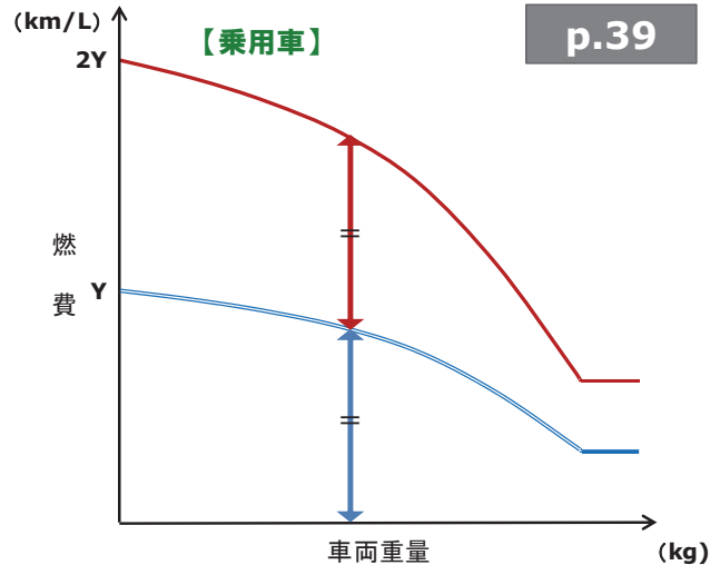
ステップレス方式の燃費基準値・燃費目標値の考え方
