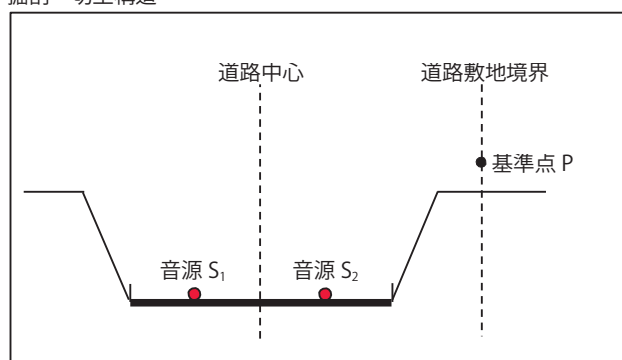
図2-2-4 掘割・切土構造
