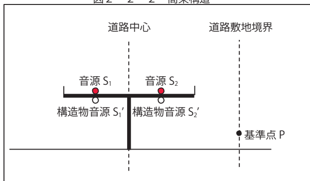
図2-2-3 盛土構造
