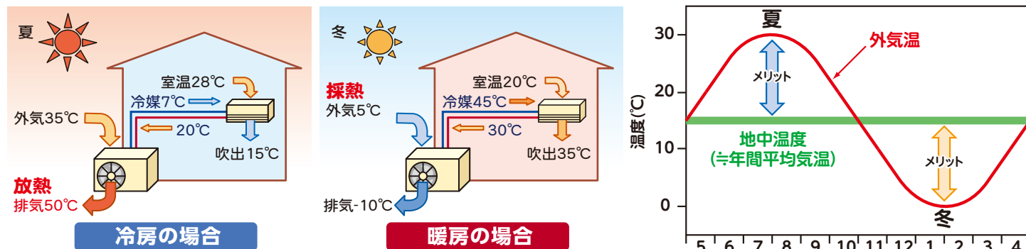
空気熱源ヒートポンプのイメージ 注) 図中の温度はイメージです。
