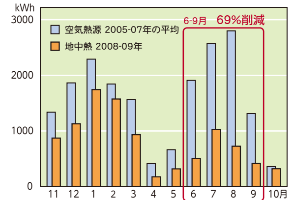
空気熱源ヒートポンプと地中熱利用ヒートポンプの消費電力の比較
