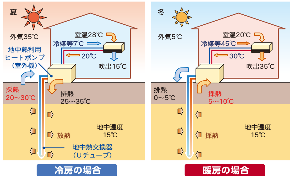
地中熱利用ヒートポンプシステムのイメージ
