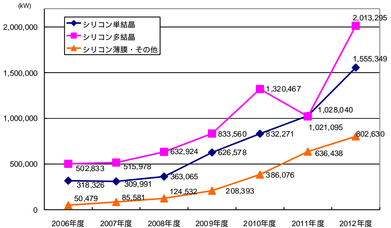
日本における太陽電池出荷量の推移
