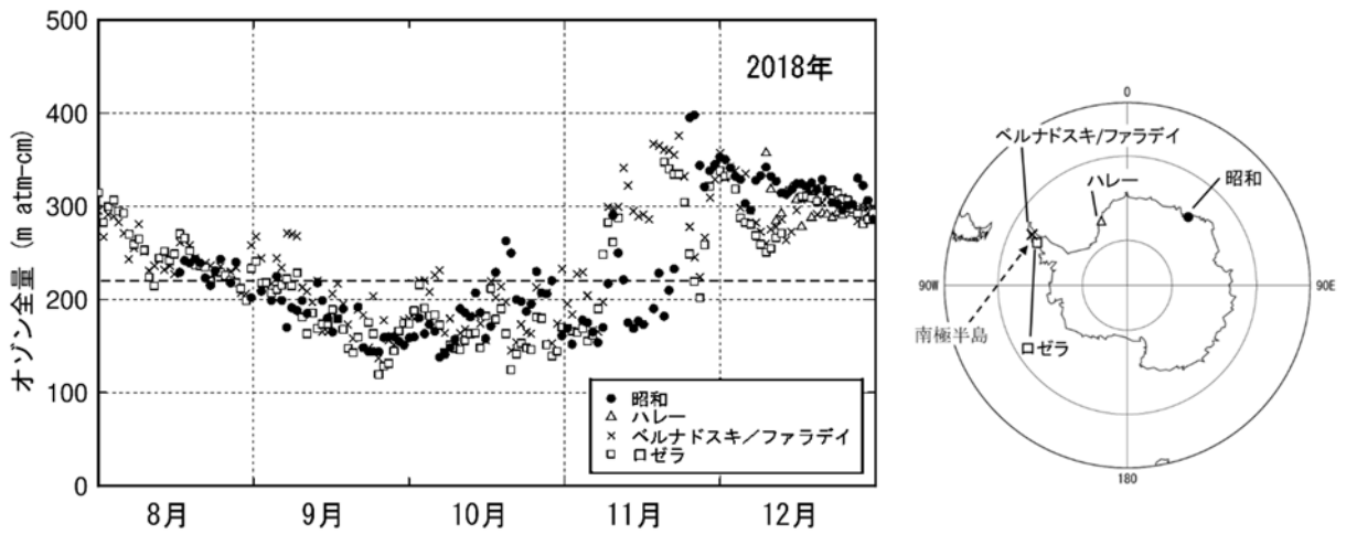
図1-資-5 南極域各国基地におけるオゾン全量の変化（2018年） （出典）気象庁 オゾン層・紫外線の年のまとめ（2018年）より
