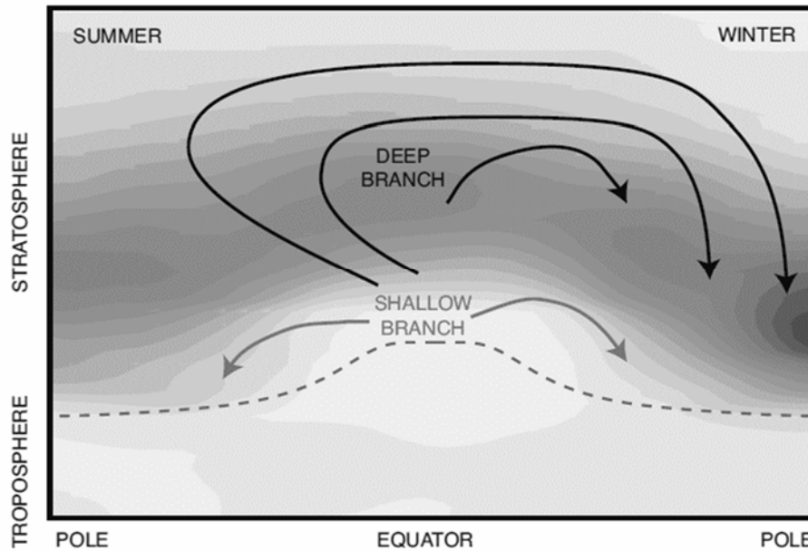
図1-資-15 ブリューワ・ドブソン循環のふたつの経路、浅い経路（shallow branch）と深い経路（deep branch）の模式図。
