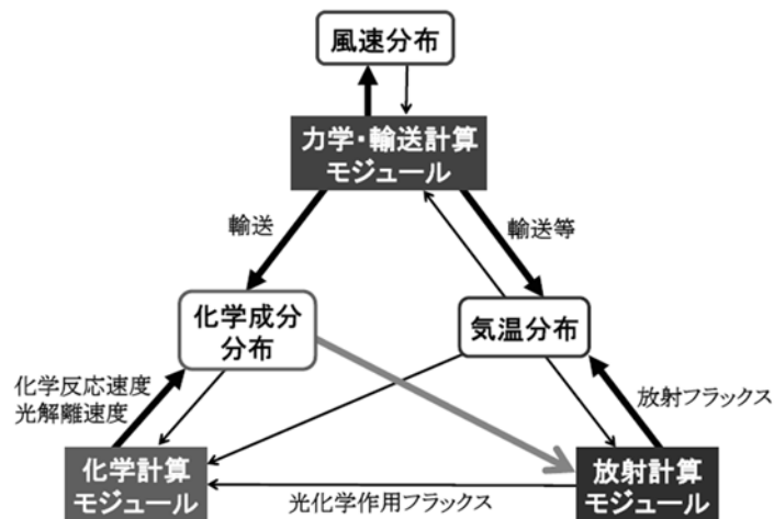
図 1-資-8 (成層圏) モデルの概念図 (出典) 永島達也ら 天気 49 巻 11 号 (2002) より
