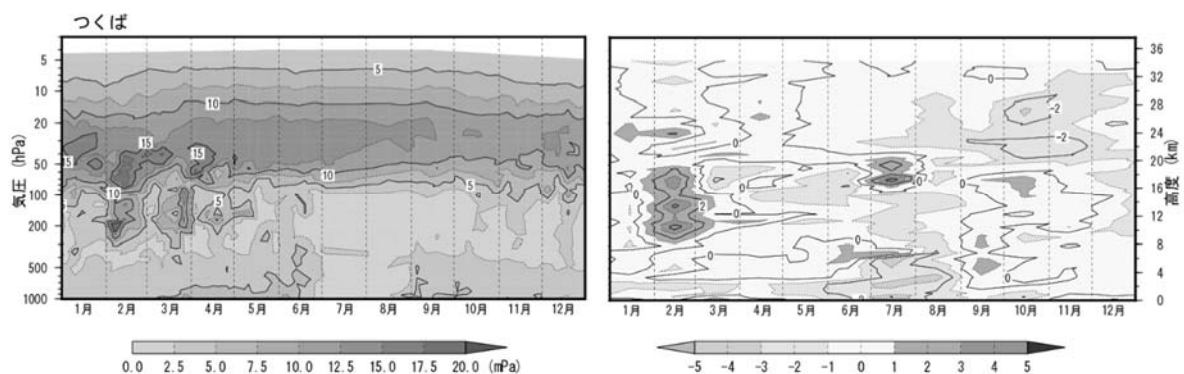
図1-資-6 つくばのオゾン分圧(左)と規格化偏差(右)の高度分布(2018年)
