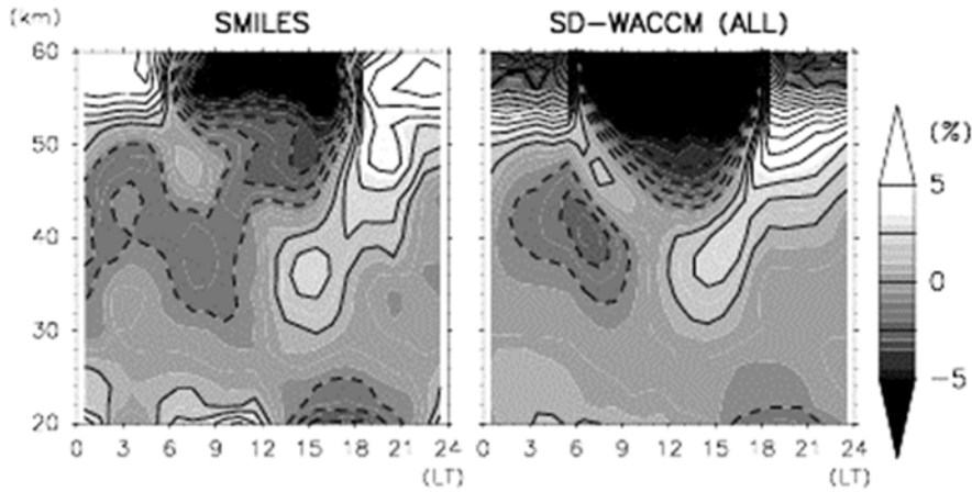
図1-資-13 熱帯（10°S-10°N）におけるオゾン量の日周期変動
