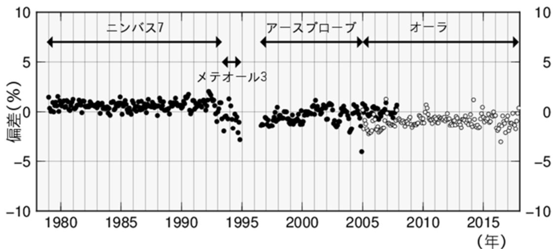
図1-資-12 衛星データと地上観測データの比較
