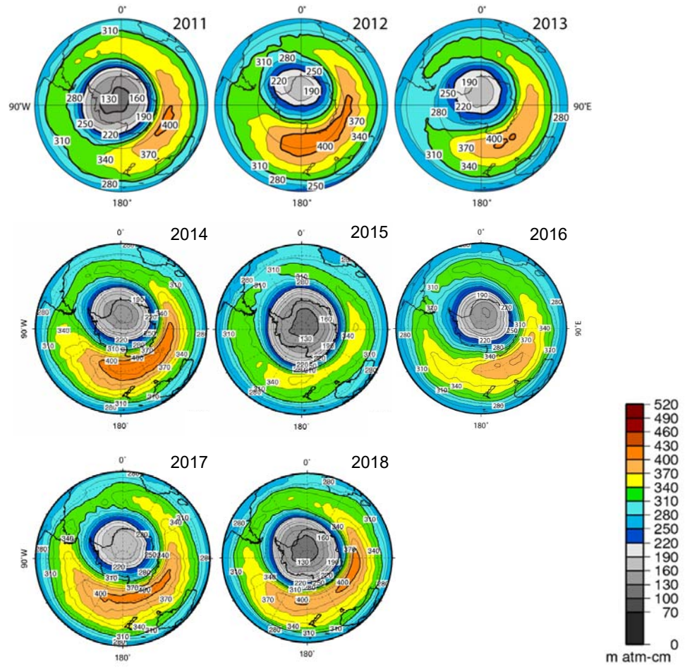
図1-資-4(3) 10月の南半球月平均オゾン全量分布図(2011~2018年) (出典) 気象庁提供データ
