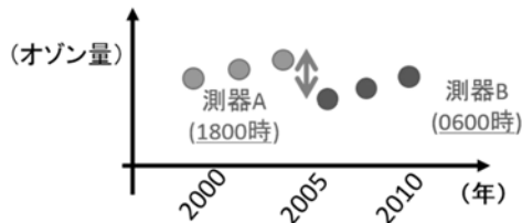
図1-資-14 オゾン量およびその長期トレンド推定に日周期変動が影響を与える例
