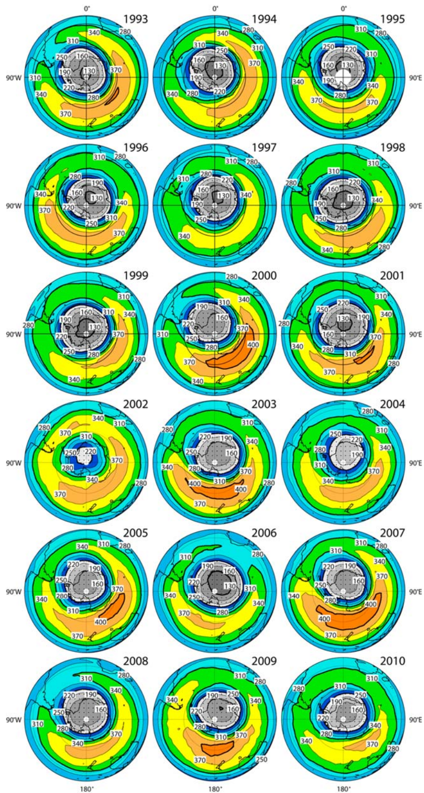
図1-資-4(2) 10月の南半球月平均オゾン全量分布図(1993~2010年) (出典) 気象庁提供データ
