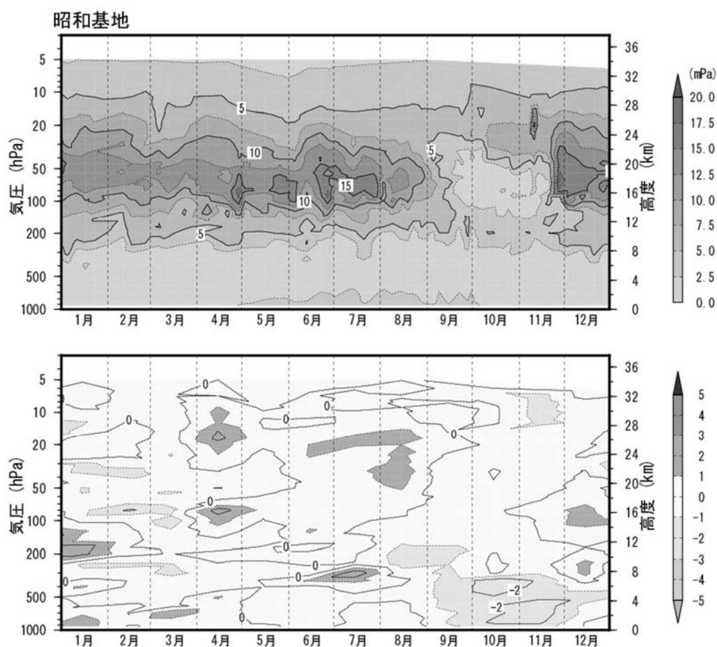
図1-資-7 南極昭和基地のオゾン分圧（上）と規格化偏差（下）の高度分布（2018年）
