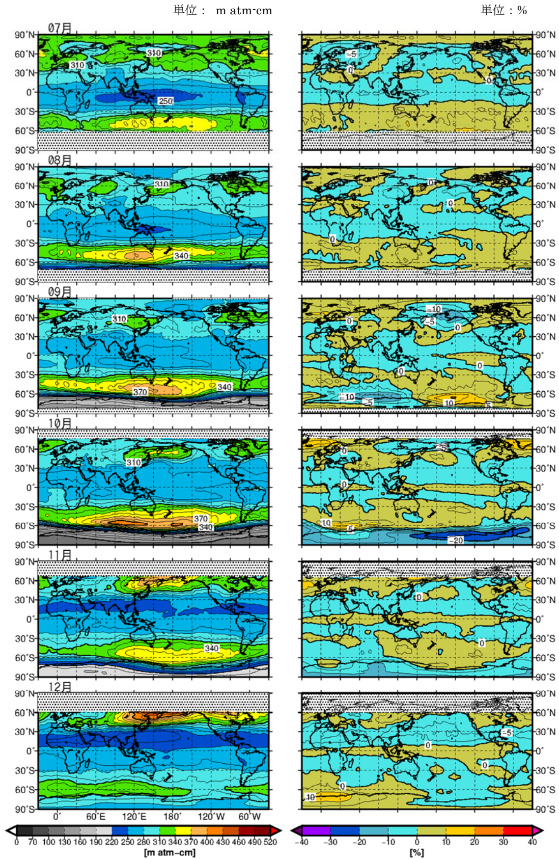
図1-資-3(2) 月平均オゾン全量・偏差(%)の地球規模の分布図(2018年7~12月)
