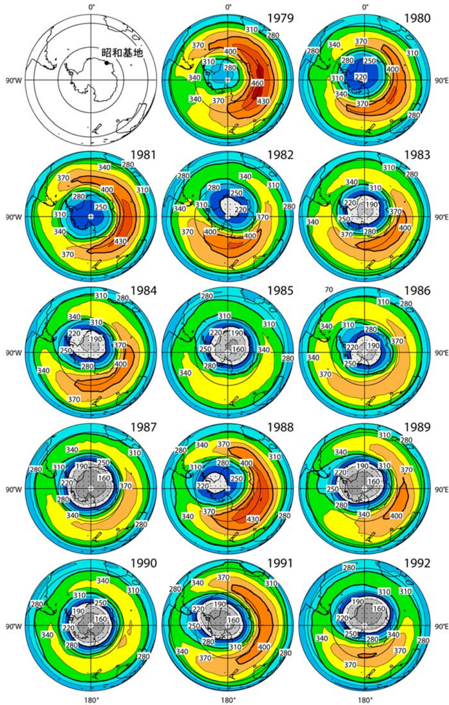
図1-資-4(1) 10月の南半球月平均オゾン全量分布図（1979～1992年） (出典) 気象庁提供データ
