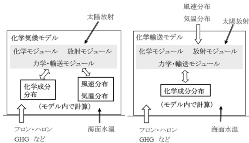
図1-資-9 化学気候モデルと化学輸送モデルの入力変数と予報変数の違い
