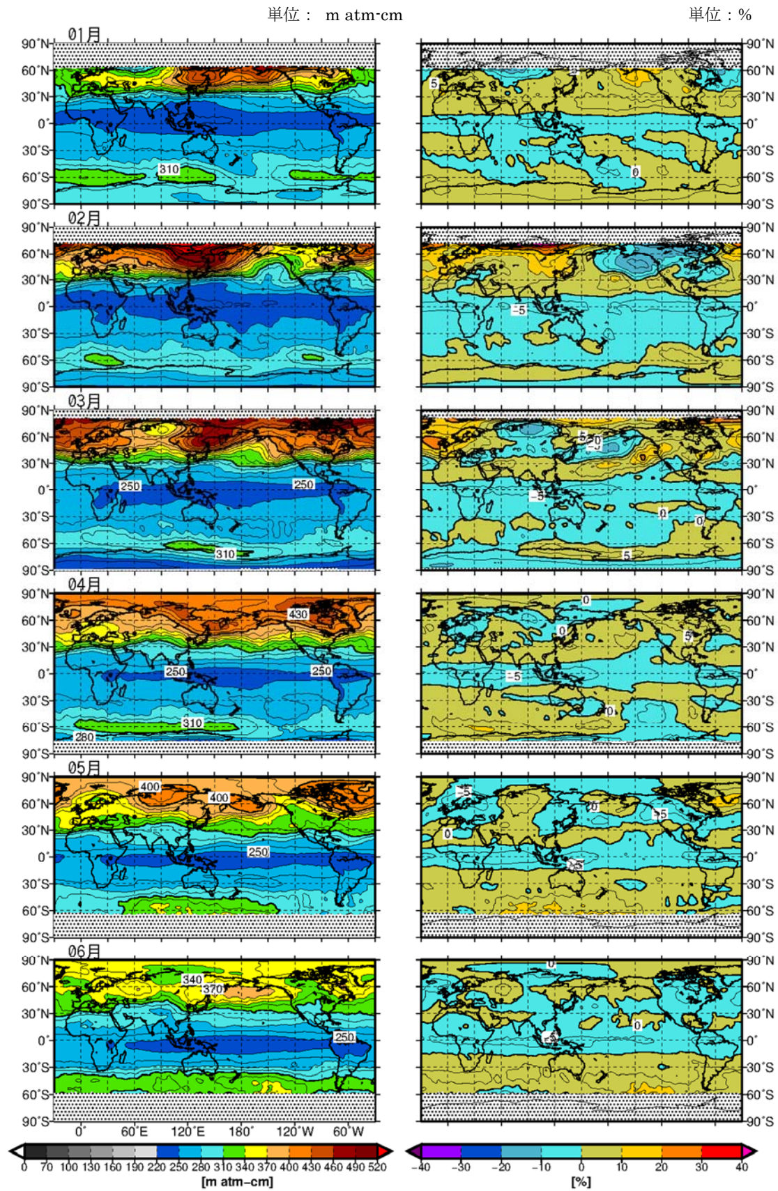
図1-資-3(1) 月平均オゾン全量・偏差(%)の地球規模の分布図(2018年1~6月) (出典) 気象庁 オゾン層・紫外線の年のまとめ(2018年)より
