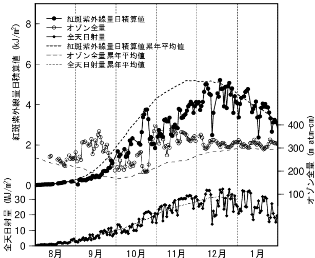
図 3-3-5 南極昭和基地における紅斑紫外線量日積算値、オゾン全量、全天日射量日積算値の推移（2019年8～1月）
