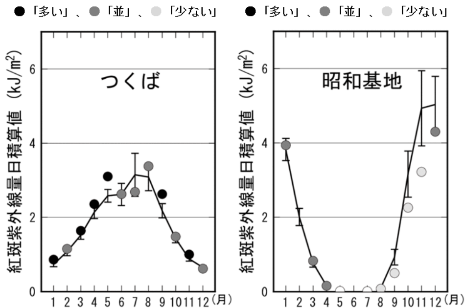
図3-3-7 2019年における紅斑紫外線量日積算値の月平均値
