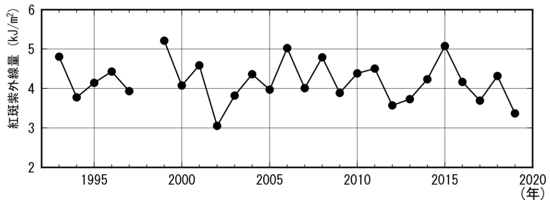
図 3-3-6 1993～2019 年までの南極昭和基地における 10～1 月平均紅斑紫外線量日積算値の経年変化
