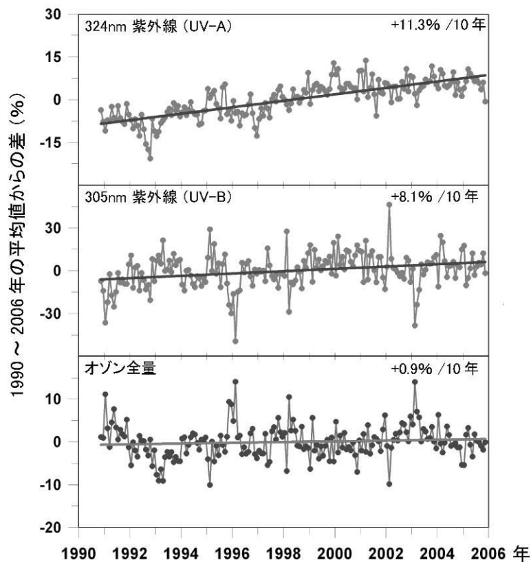
図 3-3-2 テッサロニキ（ギリシャ）におけるオゾン全量及び紫外線量の経年変化 晴天時で太陽天頂角が 63° の条件による。直線は傾向を示す。 (出典) Scientific Assessment of Ozone Depletion: 2006 (WMO, 2007)
