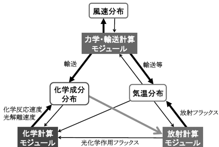
図 1-資-8 (成層圏) モデルの概念図 (出典) 永島達也ら 天気 49 巻 11 号 (2002)
