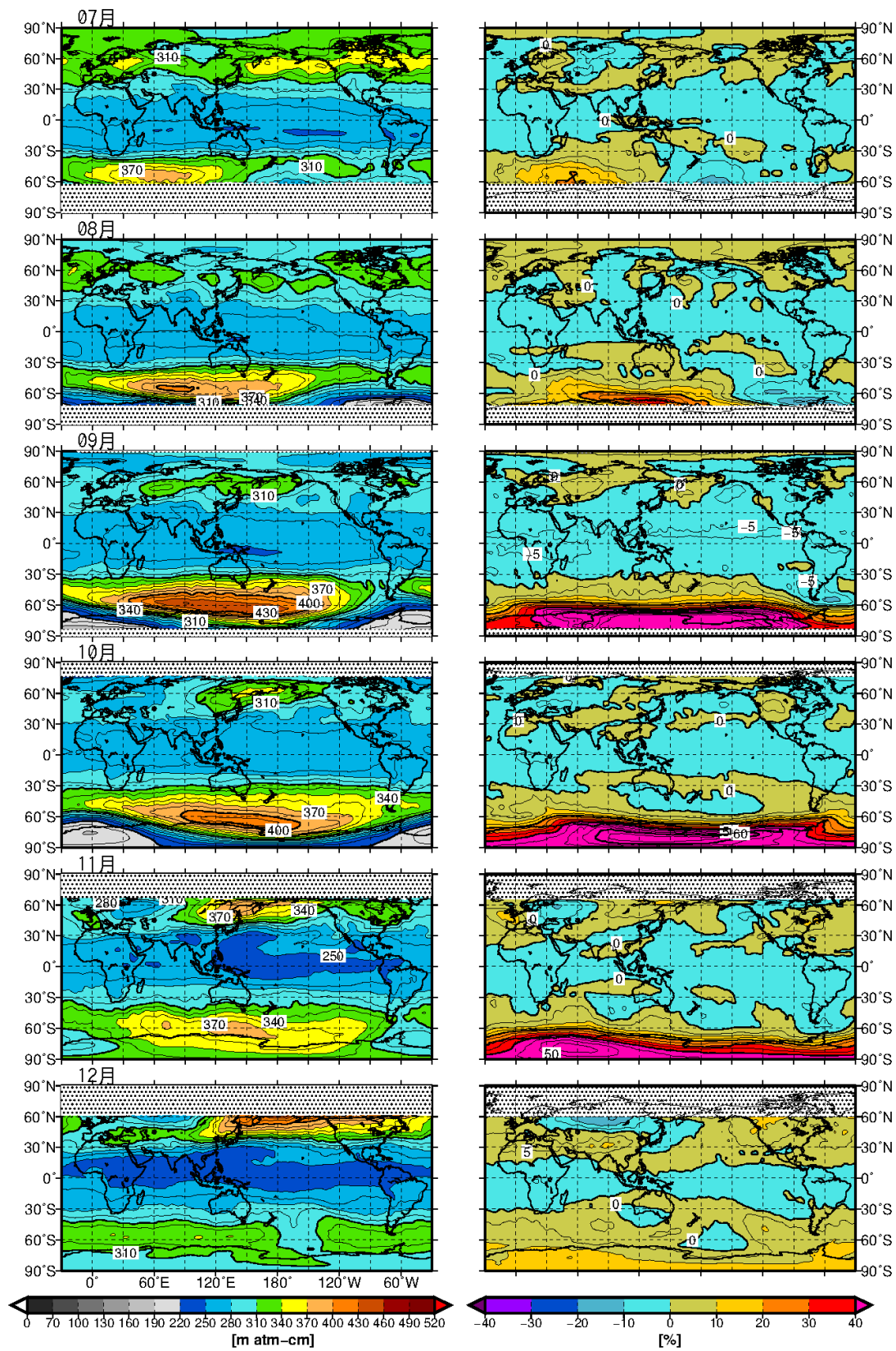
図1-資-3(2) 月平均オゾン全量・偏差(%)の地球規模の分布図(2019年7~12月)
