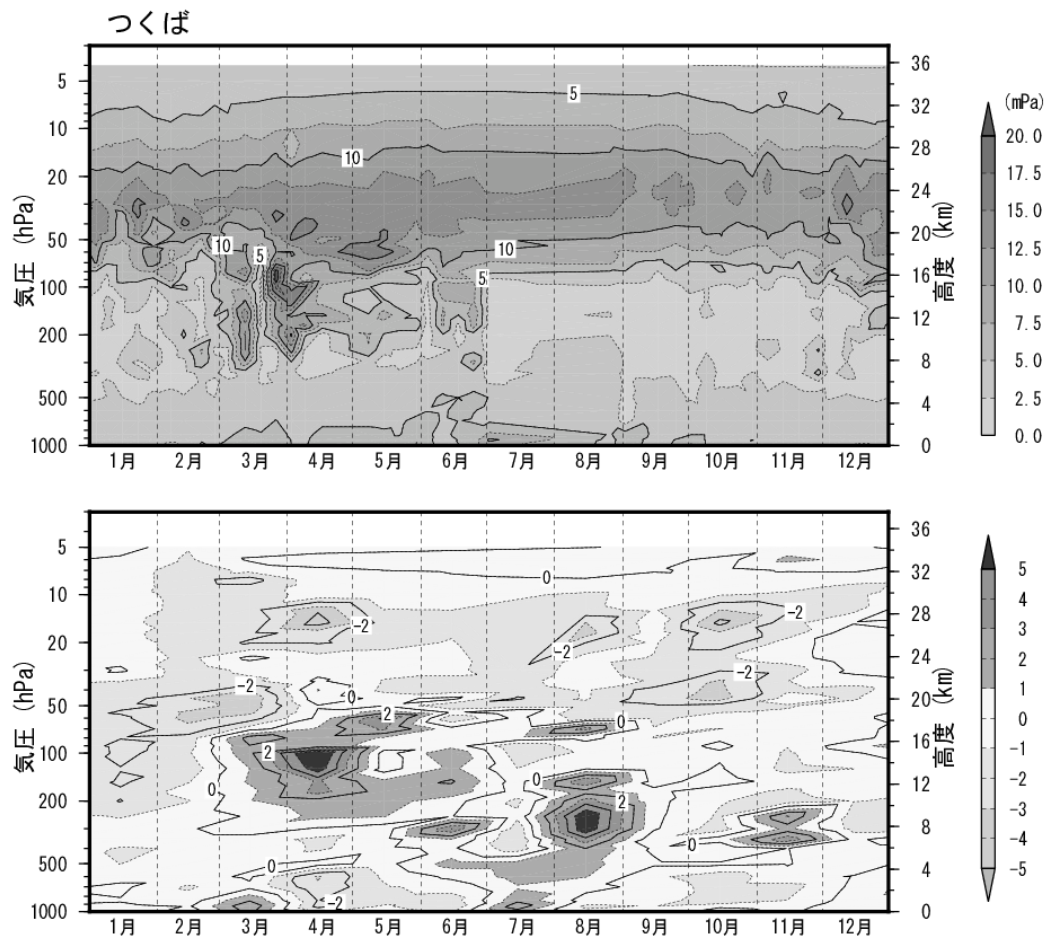
図1-資-6 つくばのオゾン分圧（左）と規格化偏差（右）の高度分布（2019年） つくばのオゾンゾンデ観測によるオゾン分圧・偏差の高度分布図。オゾン分圧図（左）は個々の観測値を用い、規格化偏差図（右）は月平均値から作成。 札幌と那覇のオゾンゾンデ観測は2018年1月に終了した。
