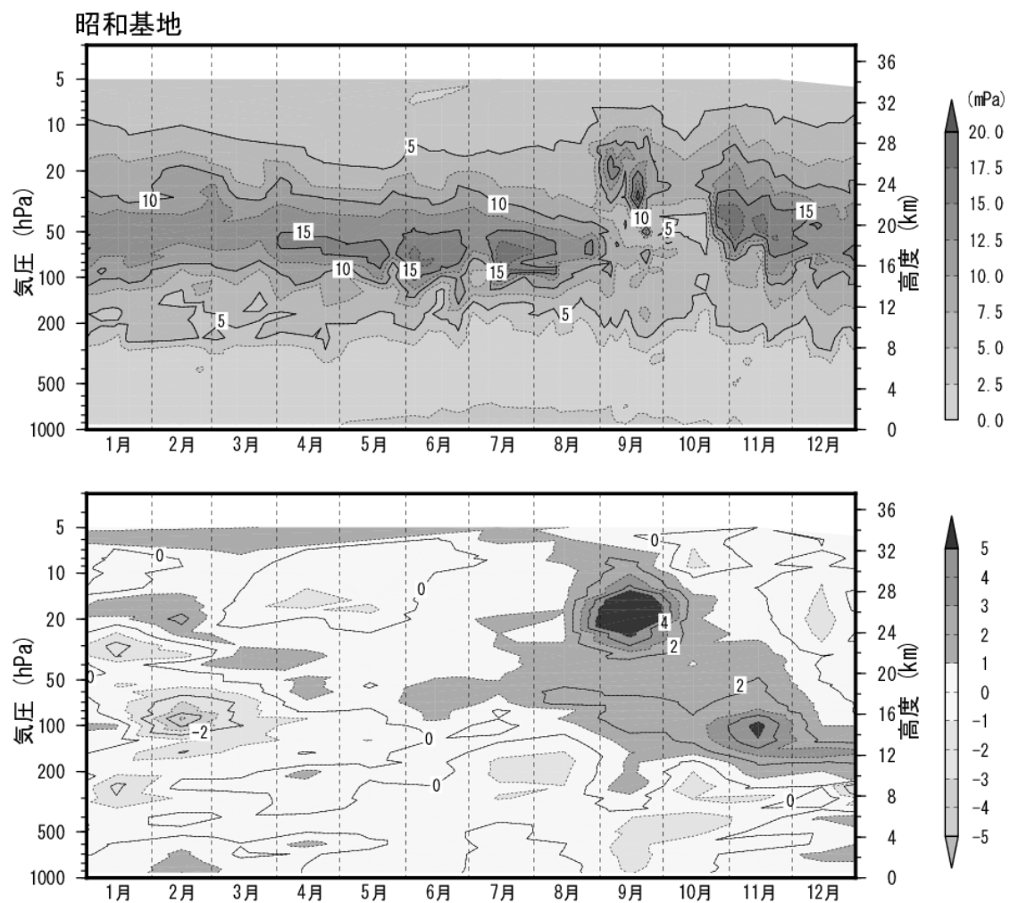
図1-資-7 南極昭和基地のオゾン分圧（上）と規格化偏差（下）の高度分布（2019年）
