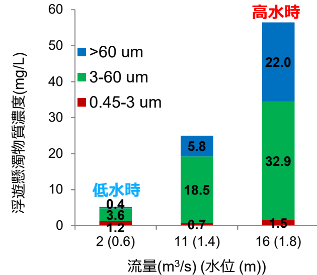
請戸川下流域（請戸川橋）での観測結果（平成26年）
