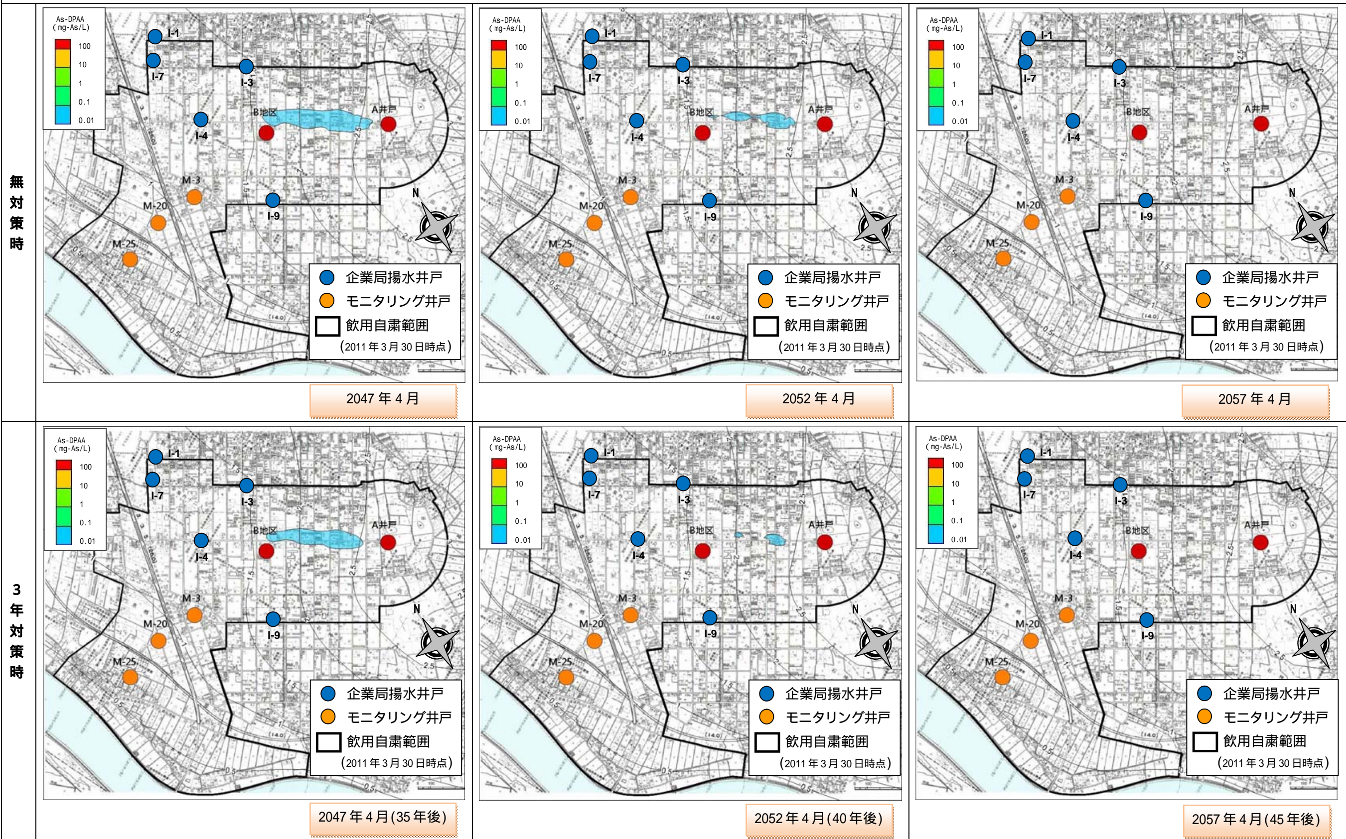
図 6.3.42 予測解析結果（無対策、3年対策）比較図：DPAA 濃度コンター図（深度 20m：4/4）
