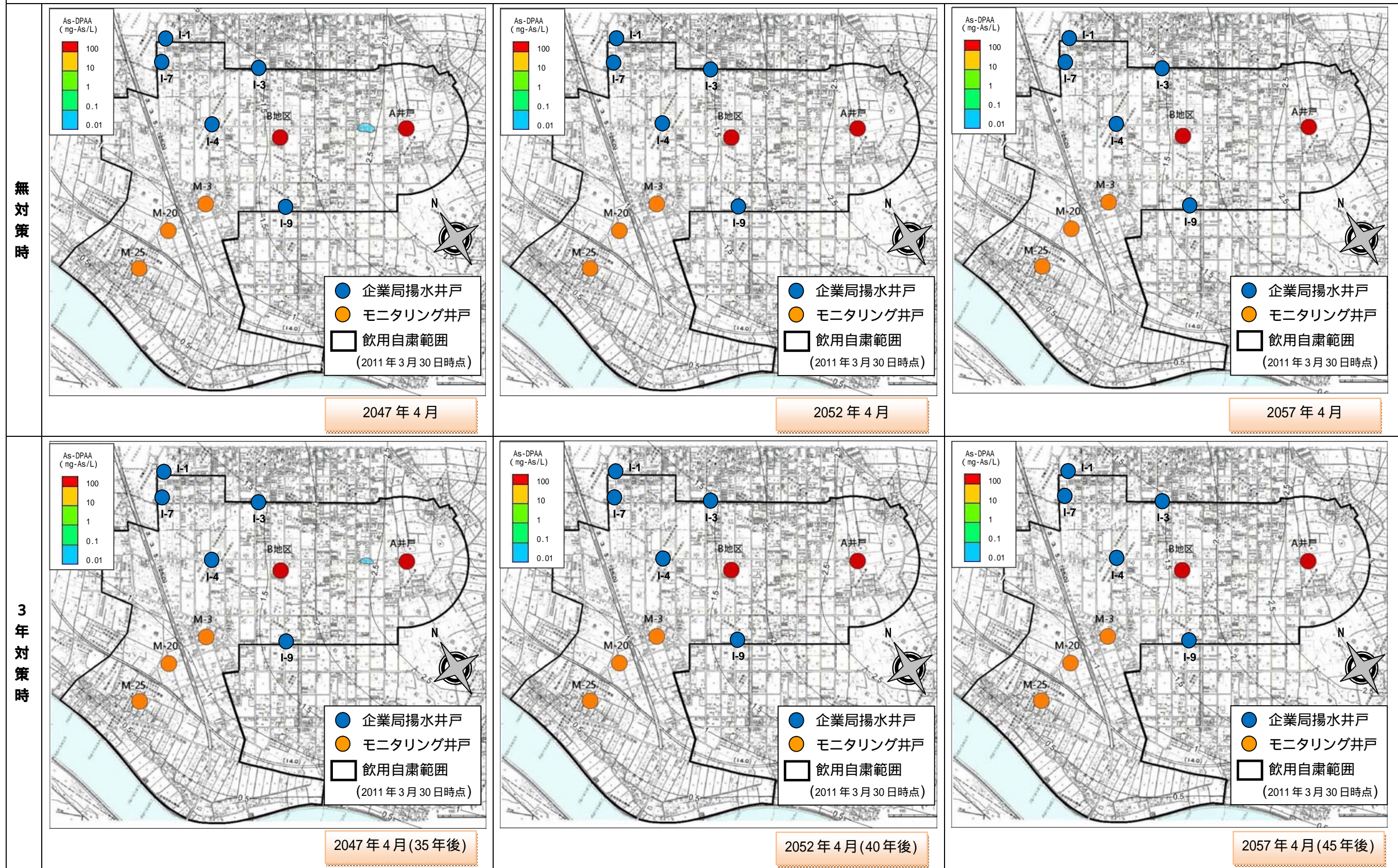
図 6.3.46 予測解析結果（無対策、3年対策）比較図：DPAA 濃度コンター図（深度 10m：4/4）
