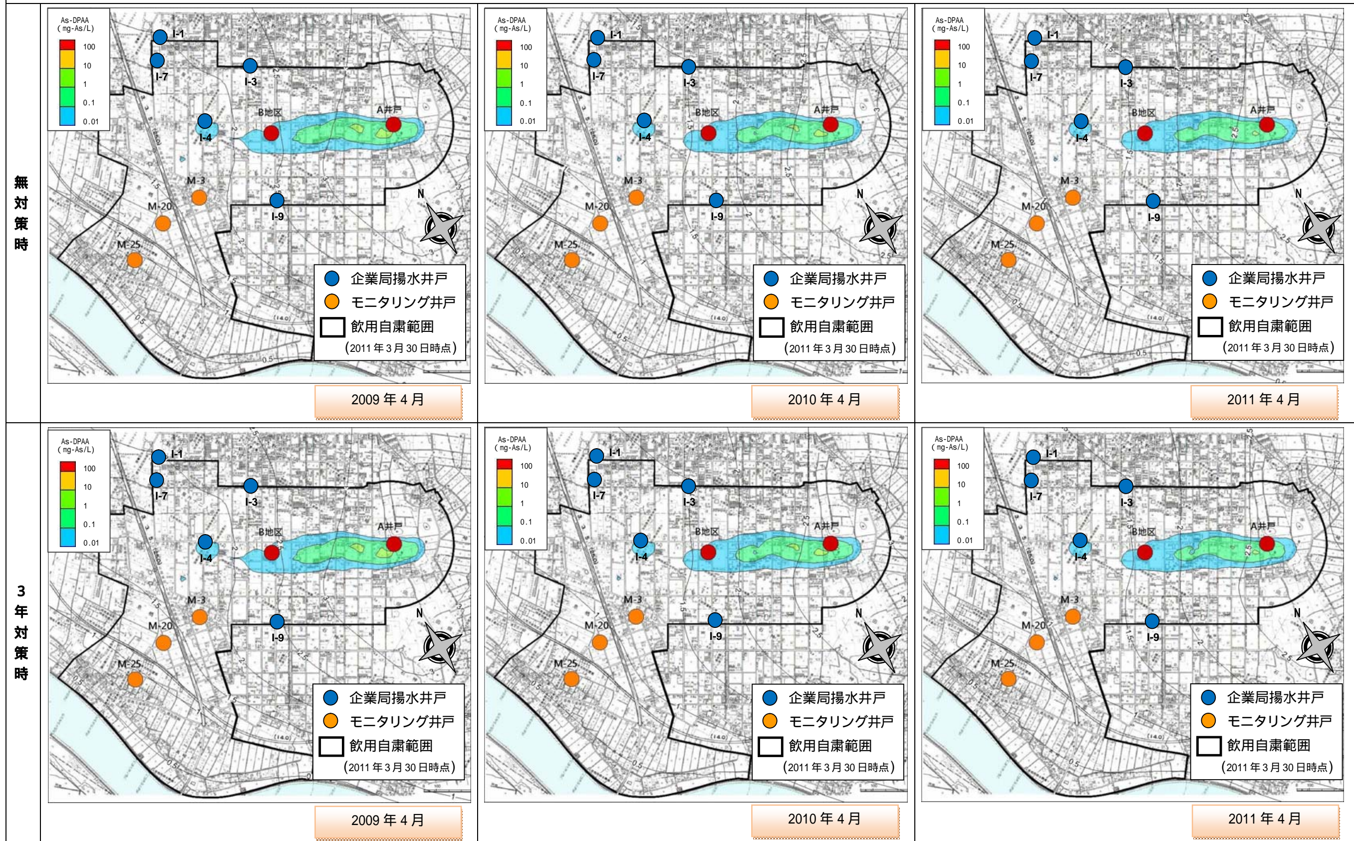
図 6.3.43 予測解析結果（無対策、3年対策）比較図：DPAA 濃度コンター図（深度 10m：1/4）
