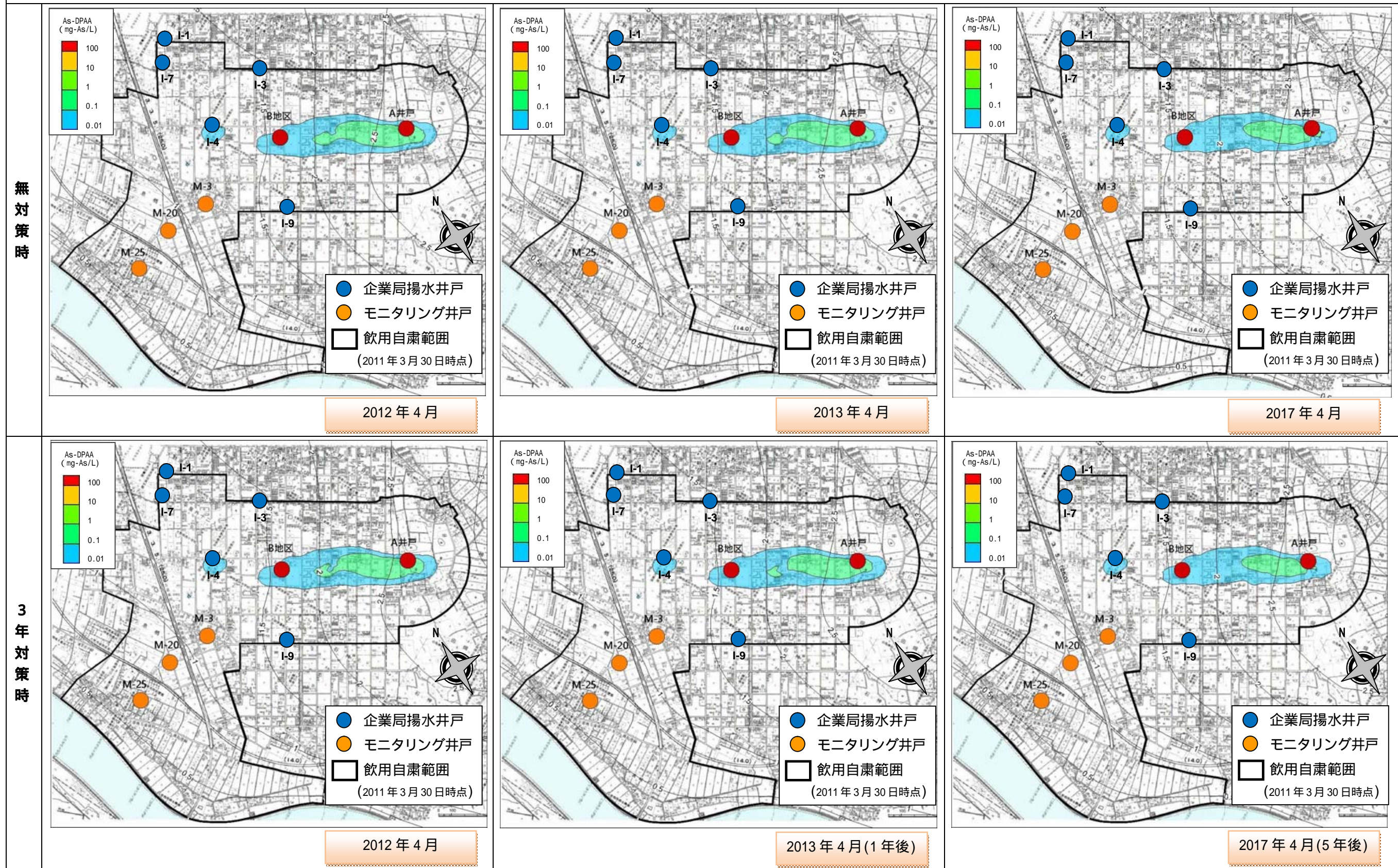
図 6.3.44 予測解析結果（無対策、3年対策）比較図：DPAA 濃度コンター図（深度 10m：2/4）
