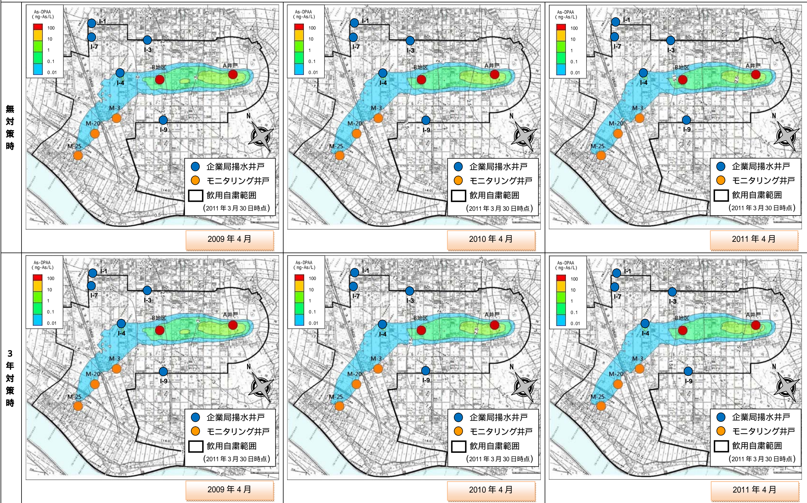
図 6.3.39 予測解析結果（無対策、3年対策）比較図：DPAA 濃度コンター図（深度 20m : 1/4）
