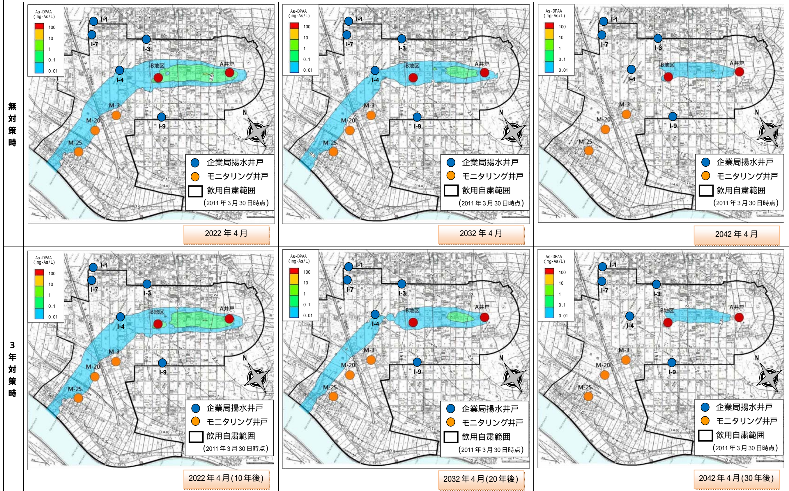
図 6.3.41 予測解析結果（無対策、3年対策）比較図：DPAA 濃度コンター図（深度 20m：3/4）
