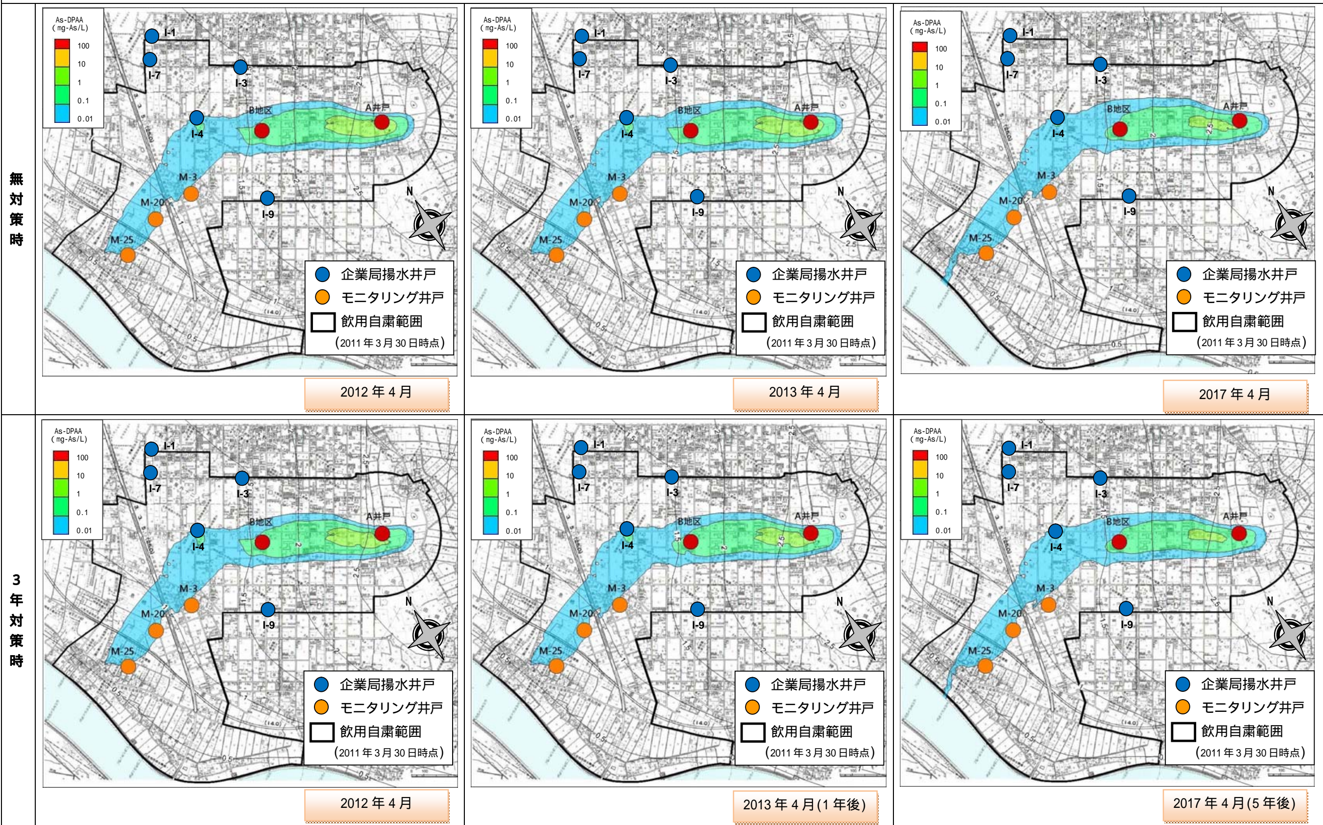
図 6.3.40 予測解析結果（無対策、3年対策）比較図：DPAA 濃度コンター図（深度 20m：2/4）
