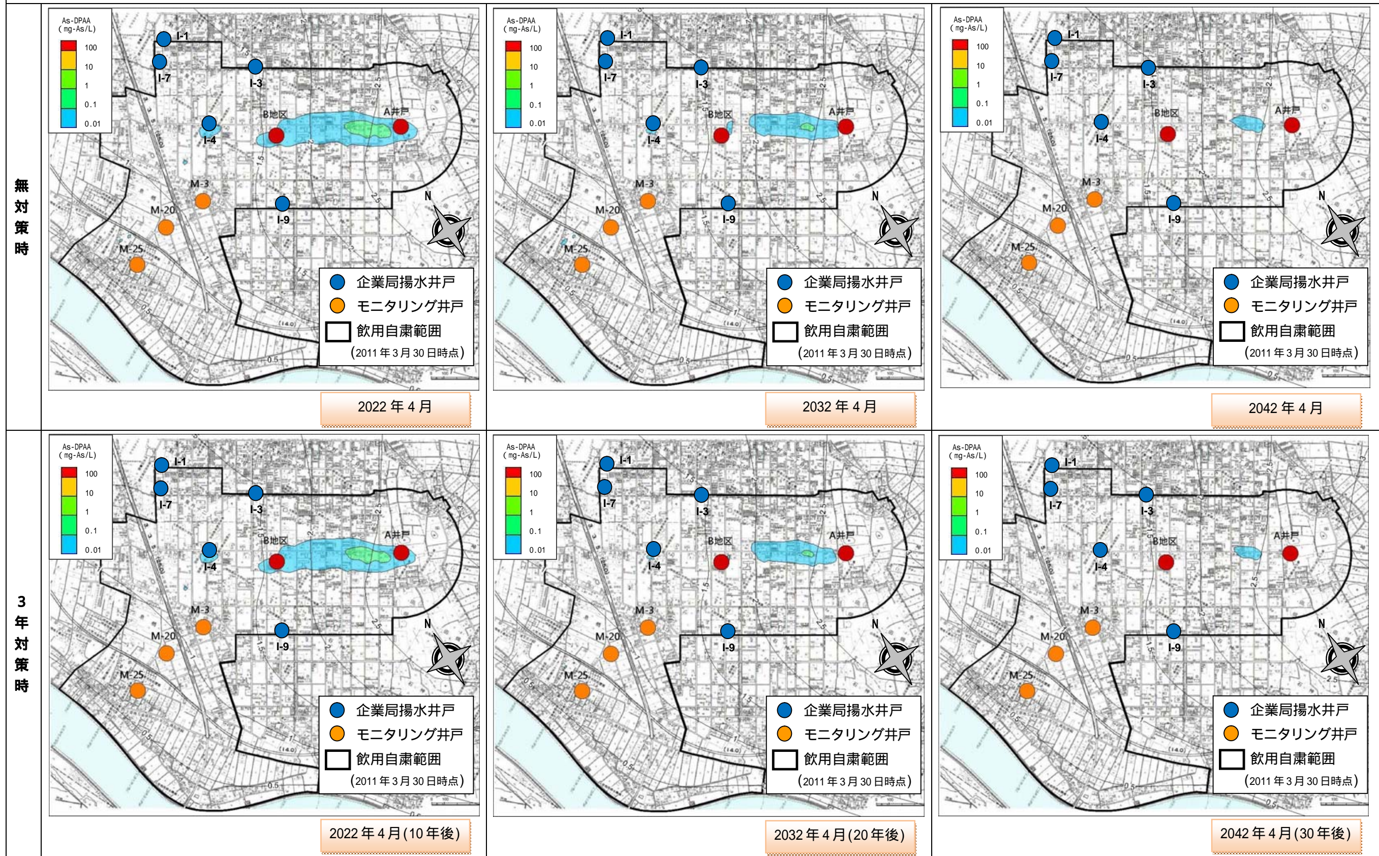
図 6.3.45 予測解析結果（無対策、3年対策）比較図：DPAA濃度コンター図（深度10m：3/4）
