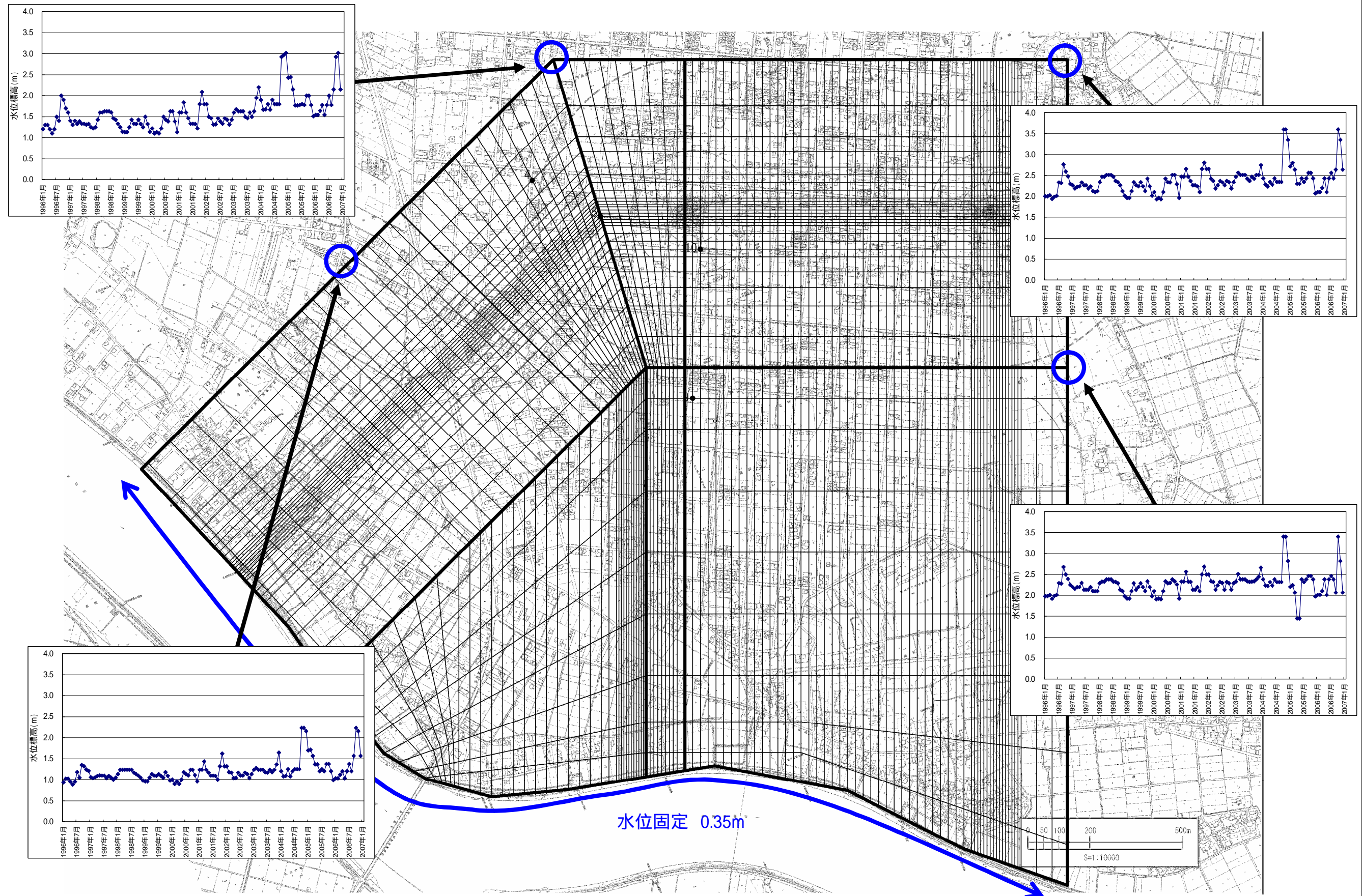
図6.4.1 ABトラック広域地下水汚染シミュレーション境界条件
