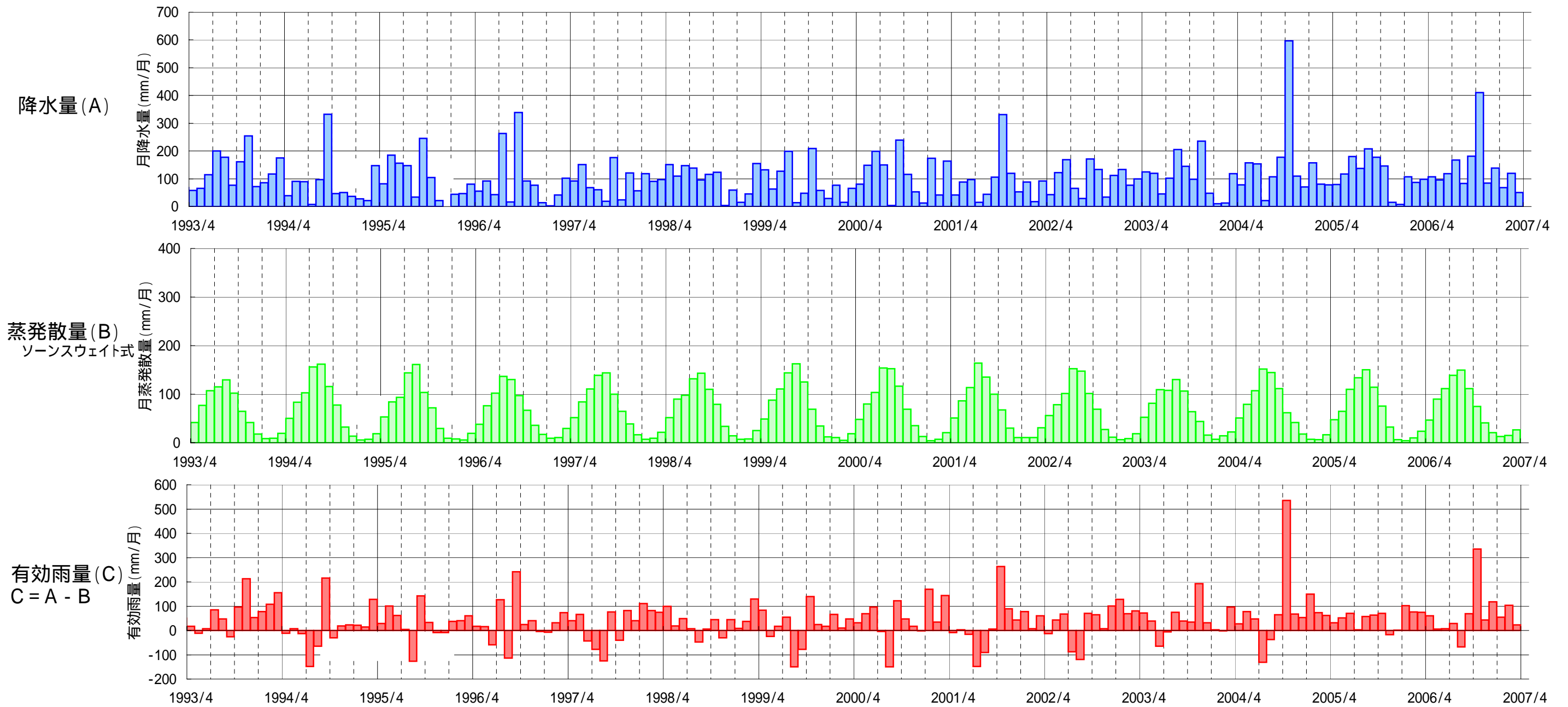
図6.4.3 降水量・蒸発散量・有効雨量(月単位)(観測地点:神栖市役所)
