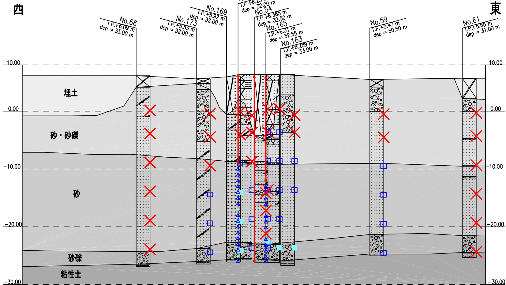
图5.2.10 初期B地区土壤・地下水DPA A污染状况断面图
