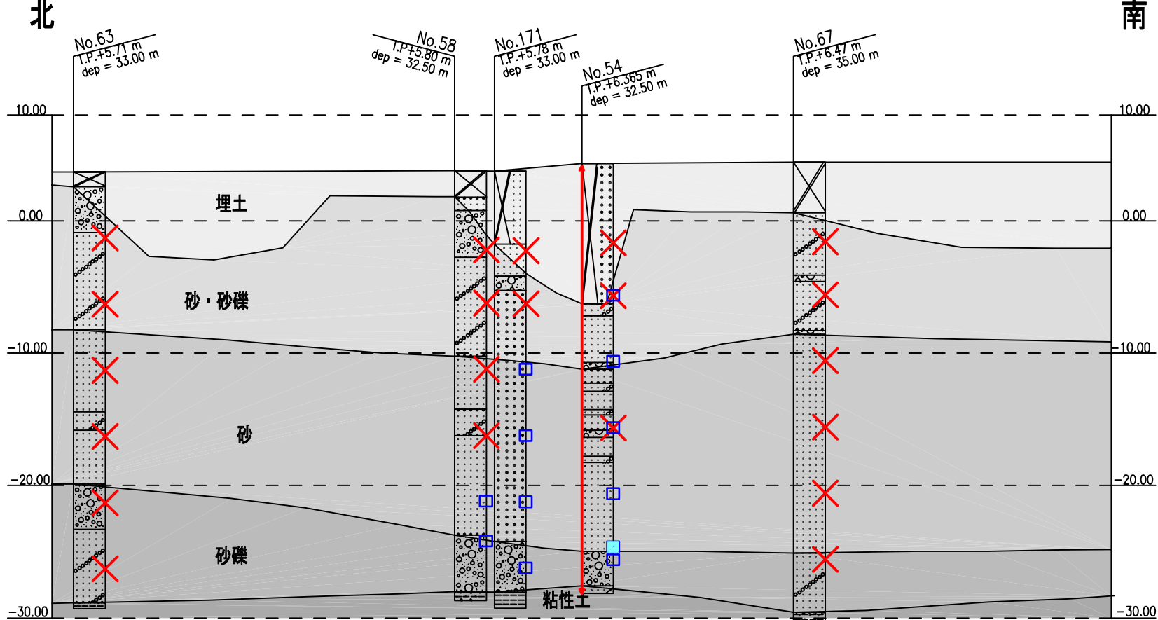
B地区南北断面图 (SH=1:2000、SV=1:400)
