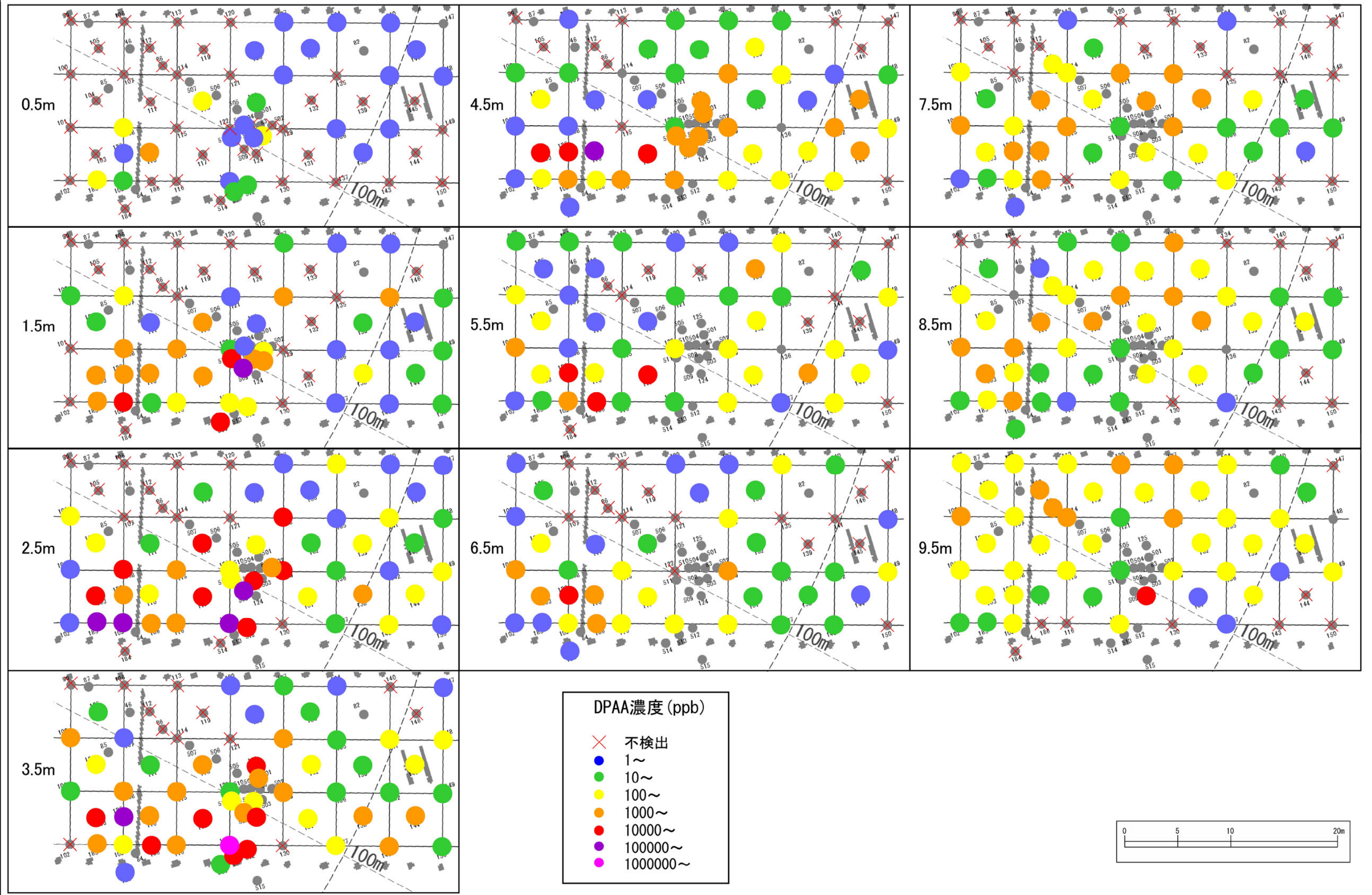
図5.2.9 初期掘削調査地点土壌DPA A汚染状況図（0.5mピッチスライス）
