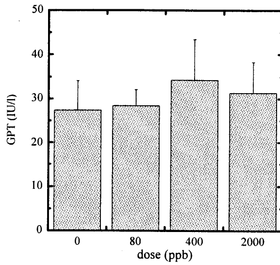
図 2 3ヶ月曝露後の各群のGPT (ALT)
