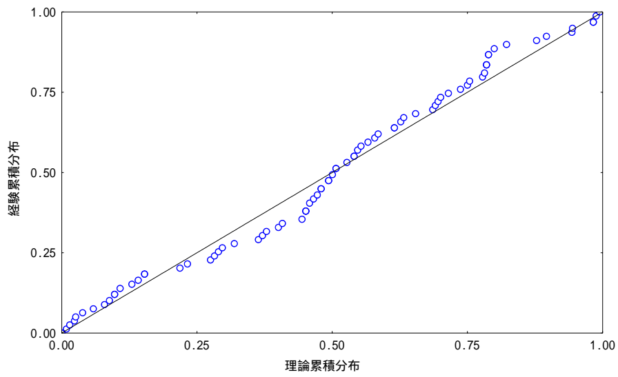
図8 トータルダイエツスタディ仮定分布のP-Pプロット
