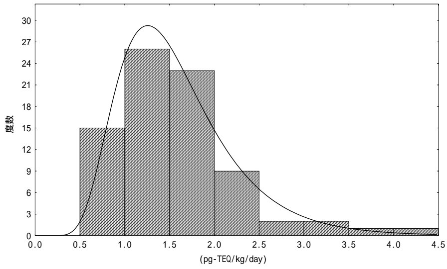
図7 トータルダイエツスタディ頻度分布への対数正規分布のあてはめ
