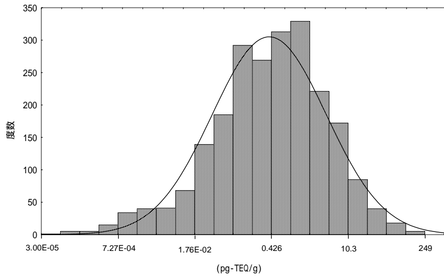
図 5 土壤中ダイオキシン類濃度頻度分布への対数正規分布のあてはめ
