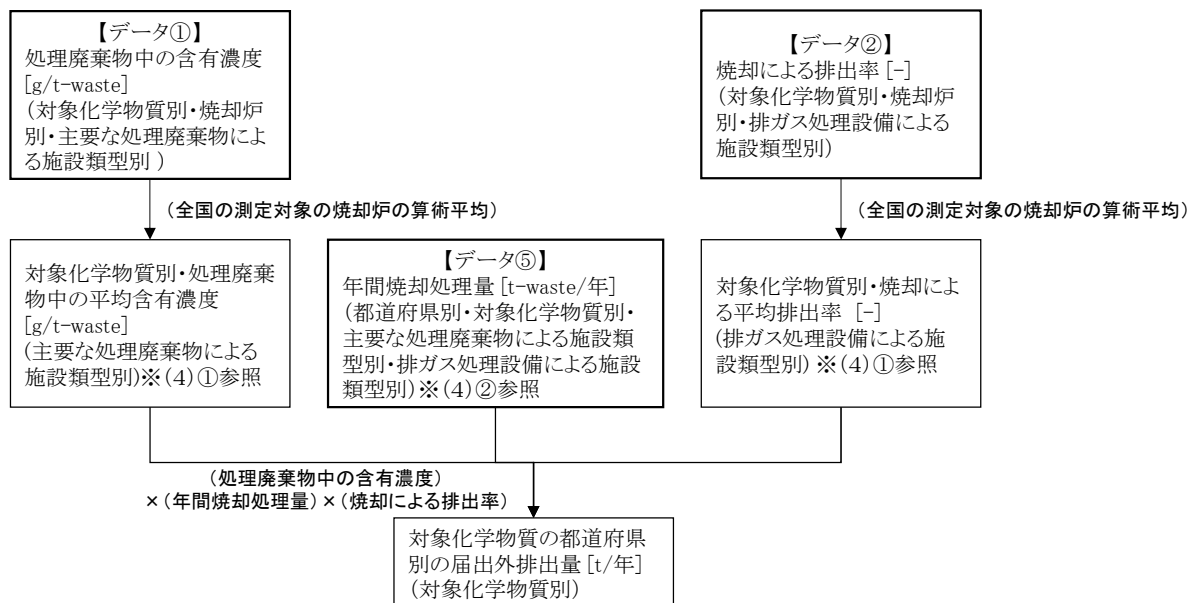
図 22-1 焼却施設に係る排出量の推計フロー(金属類)
