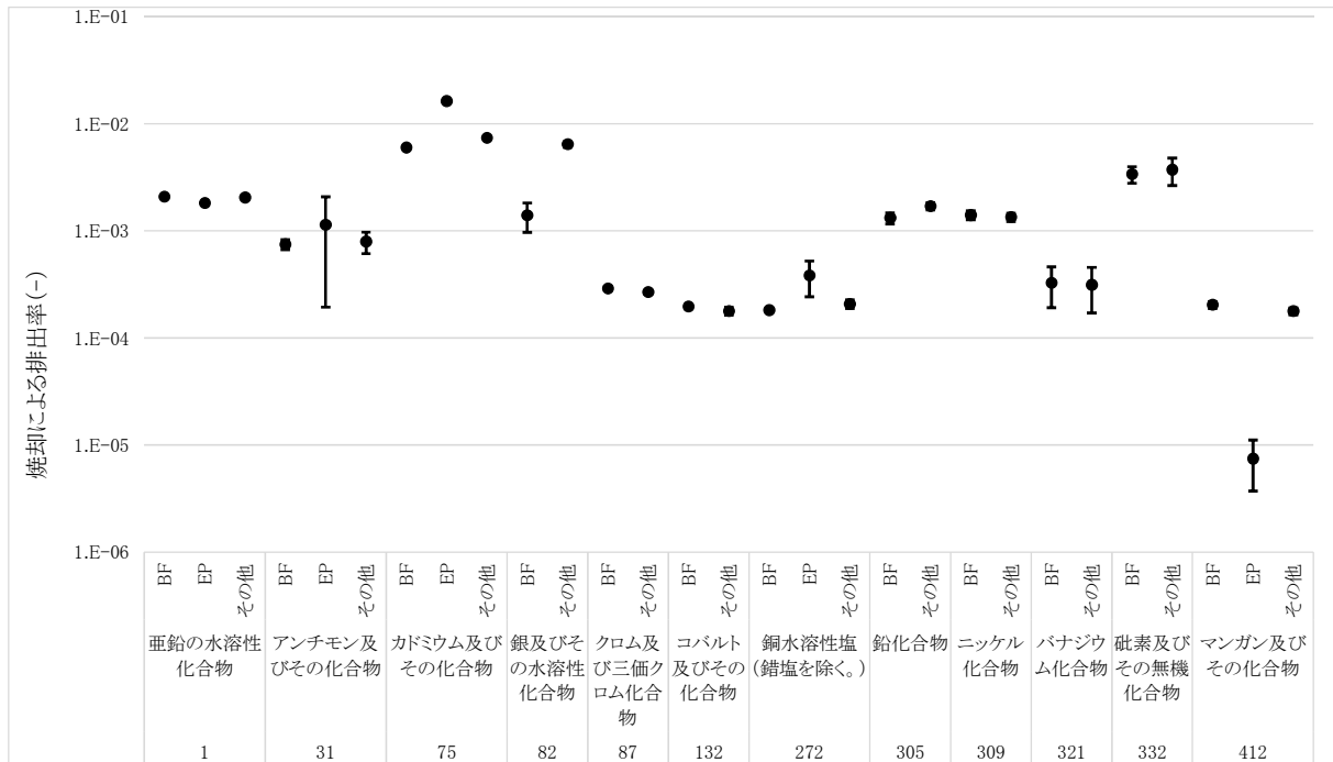
図 22-6 排ガス処理による施設類型別の焼却による排出率(金属類)
