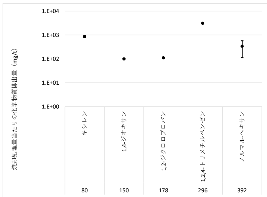
図 22-7 焼却処理量1トン当たりの化学物質排出量(有機化合物)
