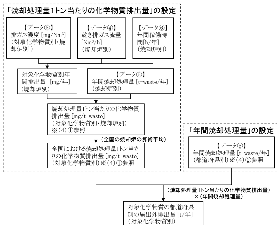
図 22-2 焼却施設に係る排出量の推計フロー(有機化合物)
