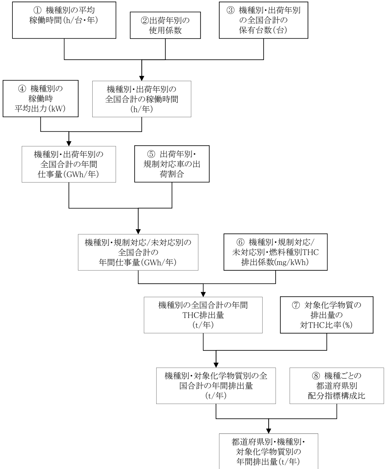
図11-39 自動車(サブエンジン式機器)に係る排出量の推計フロー
