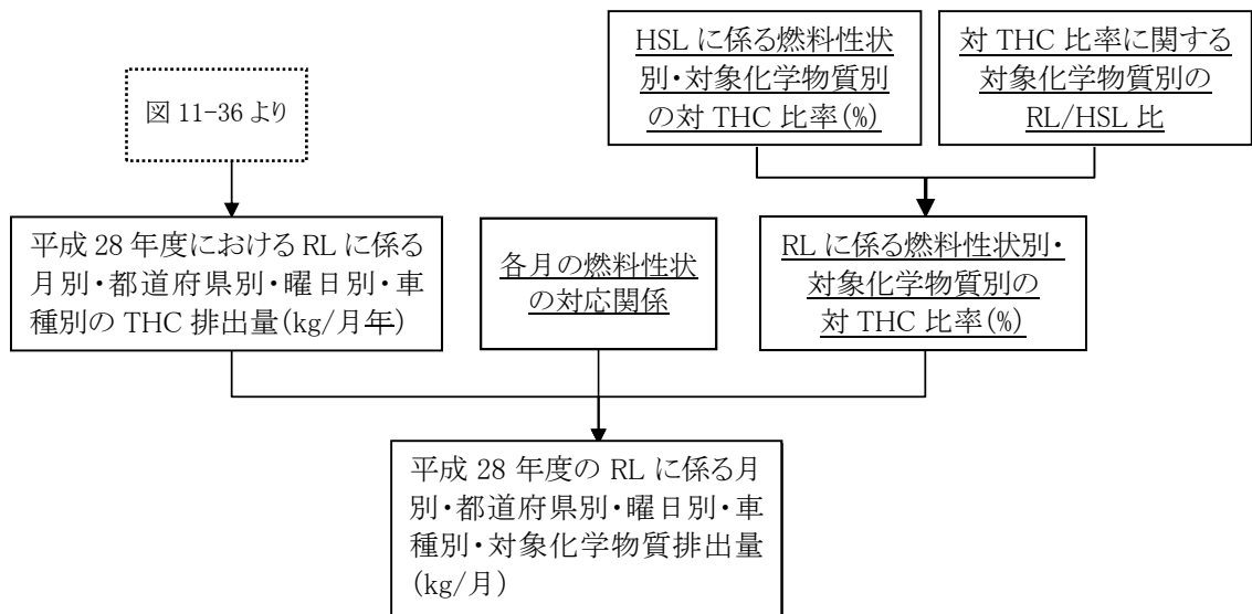
図11-38 RLに係る対象化学物質排出量の推計フロー
