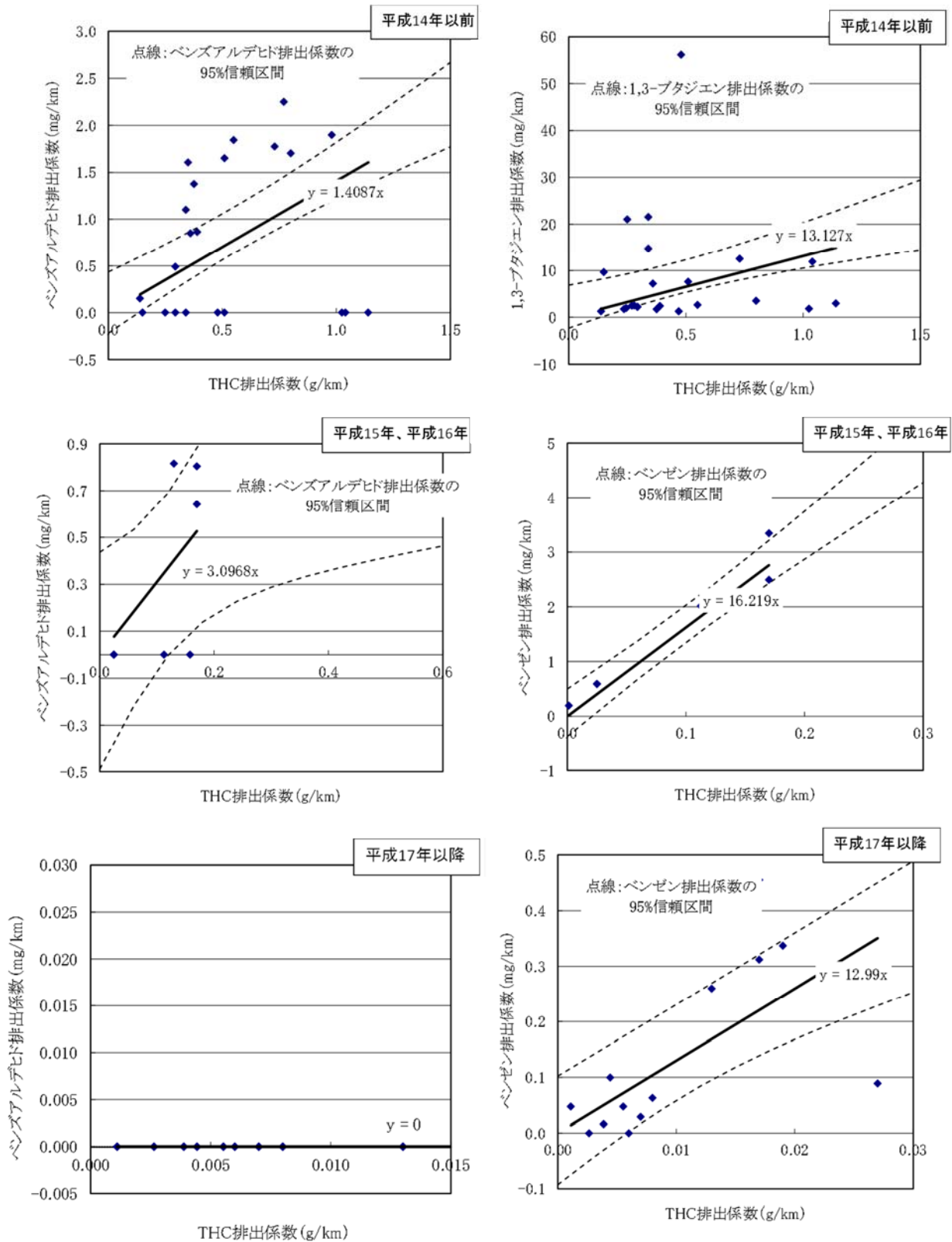
図11-43 ディーゼル自動車(ホットスタート:重量車)に係る THC 排出量と対象化学物質別排出量の比率(その 5)
