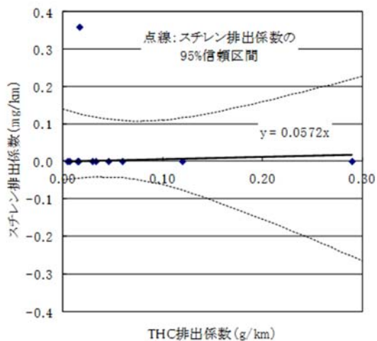
図11-41 ディーゼル自動車(ホットスタート:重量車以外(触媒あり))に係る THC 排出量と対象化学物質別排出量の比率(その1)
