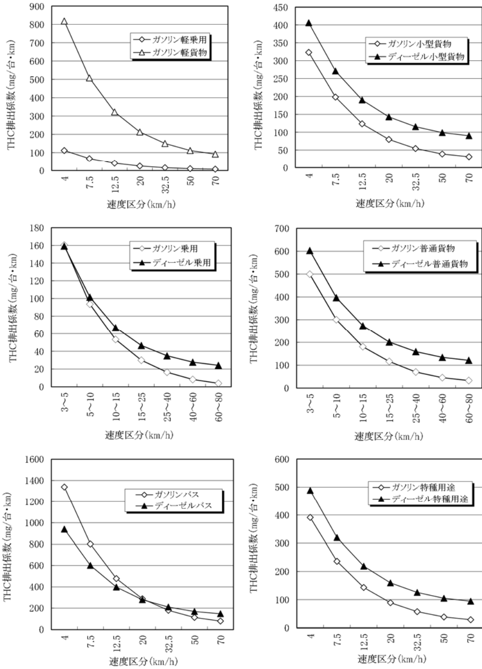
図11-13 車種別・旅行速度区分別の THC 排出係数(平成 28 年度:触媒の劣化補正後)
