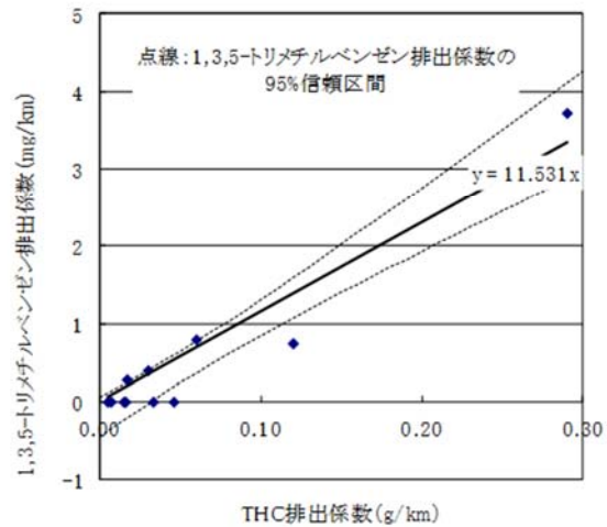
図11-41 ディーゼル自動車(ホットスタート:重量車以外(触媒あり))に係る THC 排出量と対象化学物質別排出量の比率(その1)
