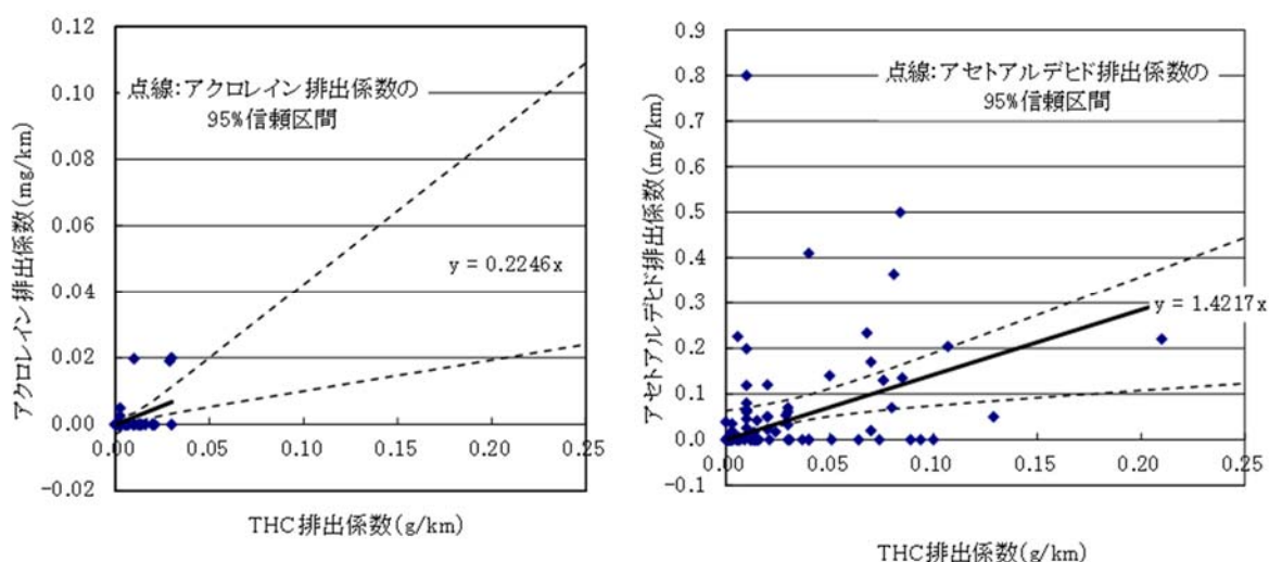
図11-40 ガソリン自動車(ホットスタート)に係る THC 排出量と対象化学物質別排出量の比率(その1)
