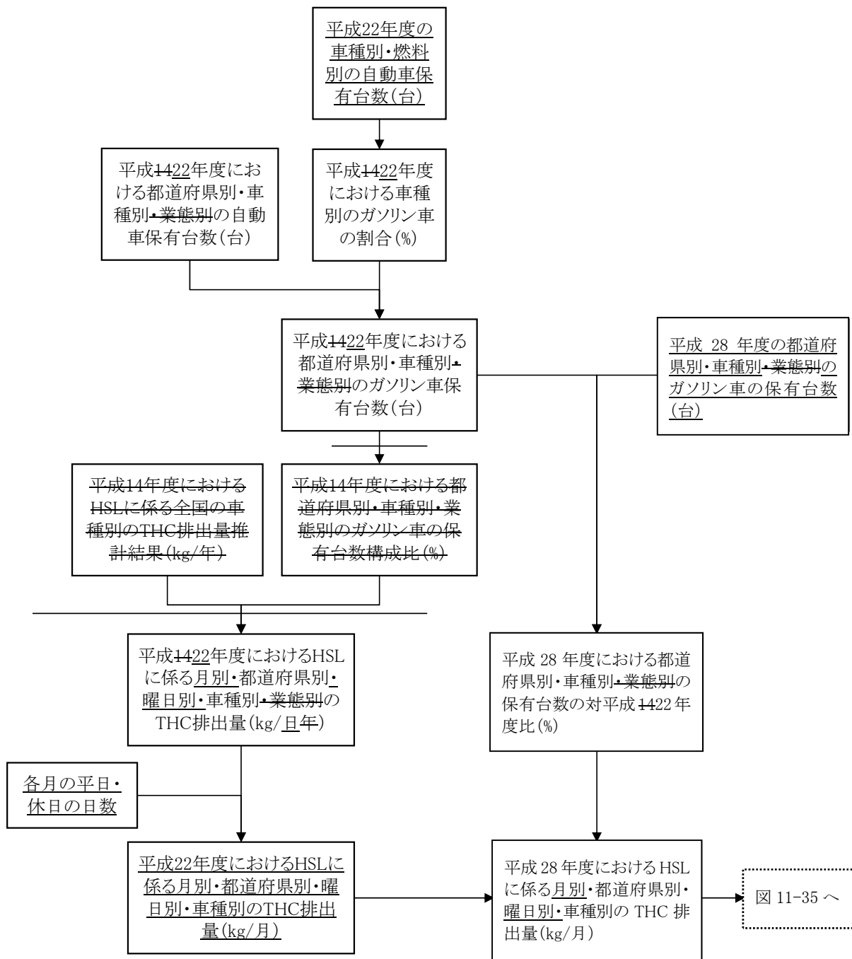
図11-35 HSLに係るTHC排出量の推計フロー
