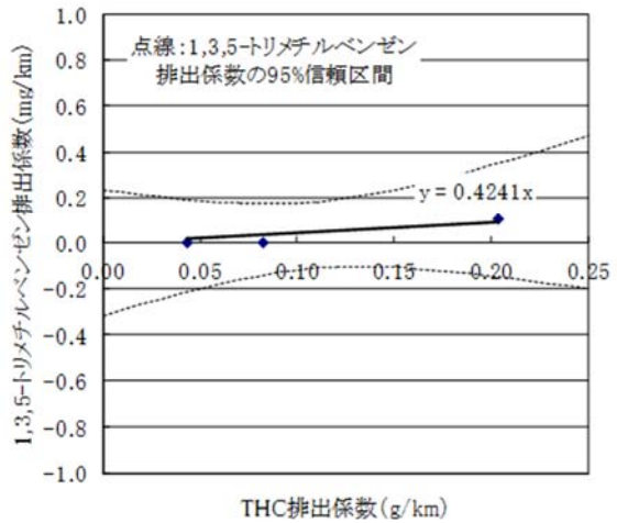
図11-42 ディーゼル自動車(ホットスタート: 重量車以外(触媒なし))に係る THC 排出量と対象化学物質別排出量の比率(その1)
