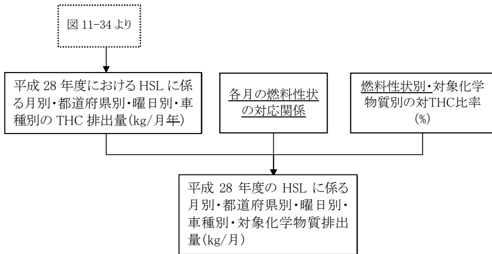
図11-36 HSL に係る対象化学物質排出量の推計フロー
