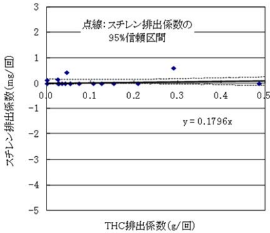
図11-45 ディーゼル自動車(コールドスタート時の増分)に係る THC 排出量と対象化学物質別排出量の比率(その1)
