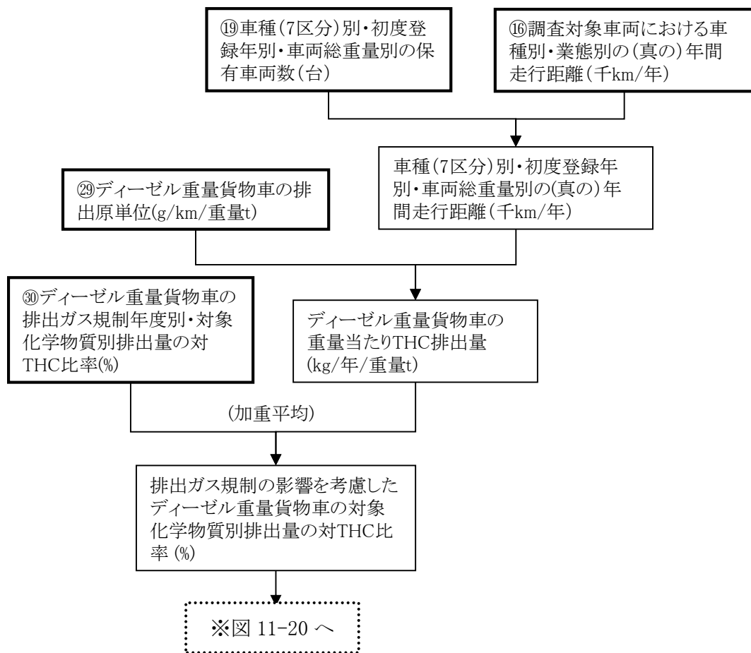
図11-19 自動車(ホットスタート)に係るディーゼル重量貨物車の対 THC 比率の設定フロー
