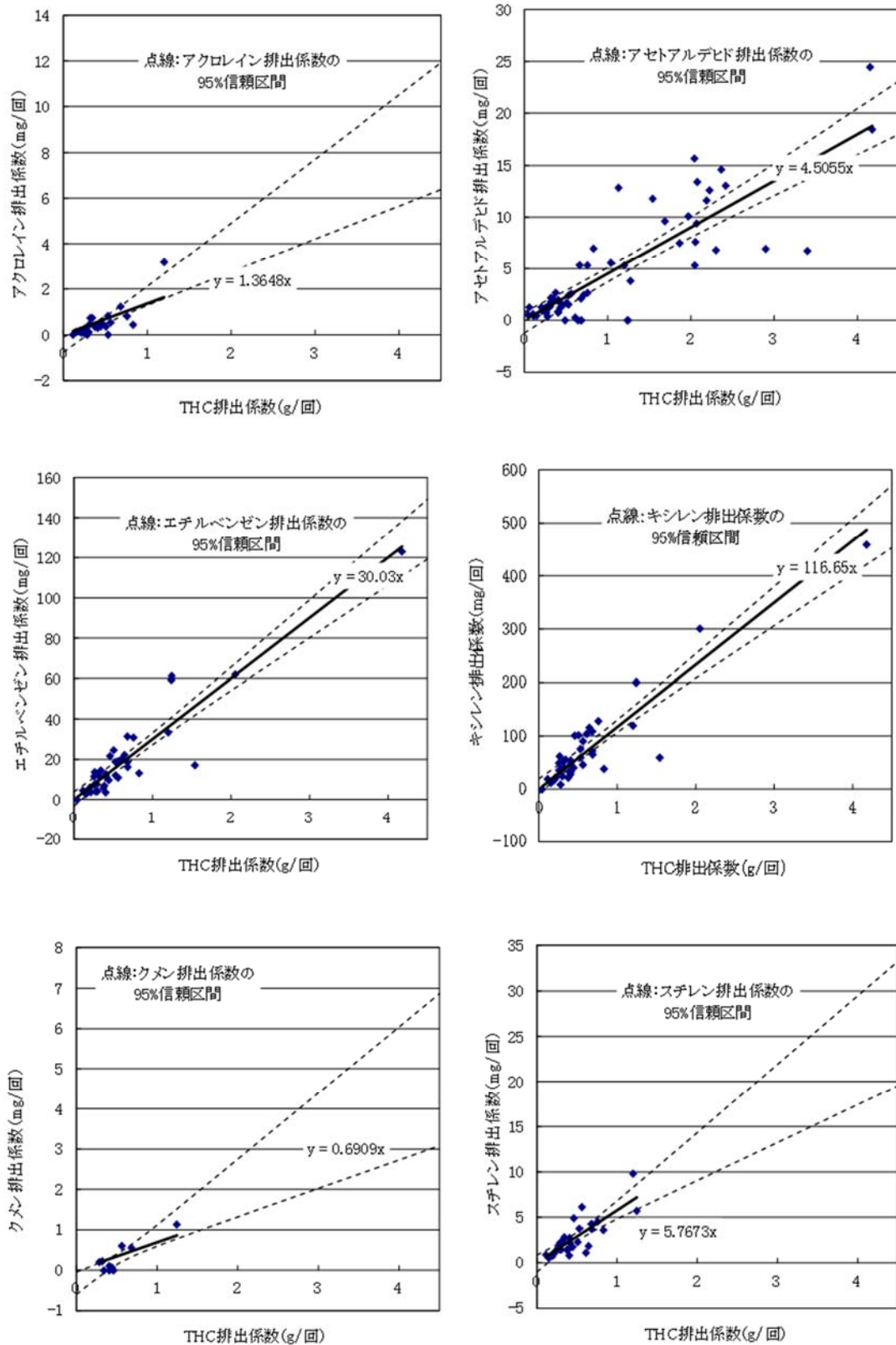
資料:環境省環境管理技術室 図11-44 ガソリン自動車(コールドスタート時の増分)に係る THC 排出量と対象化学物質別排出量の比率(その1)
