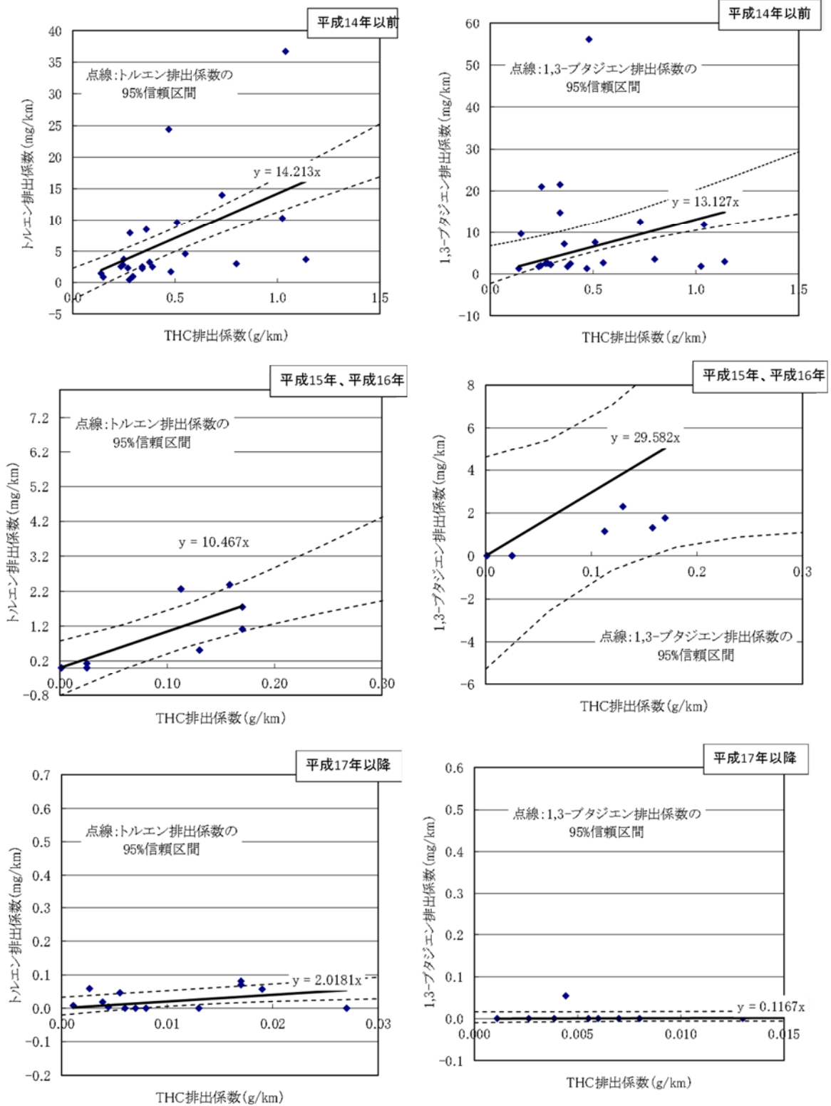
図11-43 ディーゼル自動車(ホットスタート:重量車)に係る THC 排出量と対象化学物質別排出量の比率(その4)
