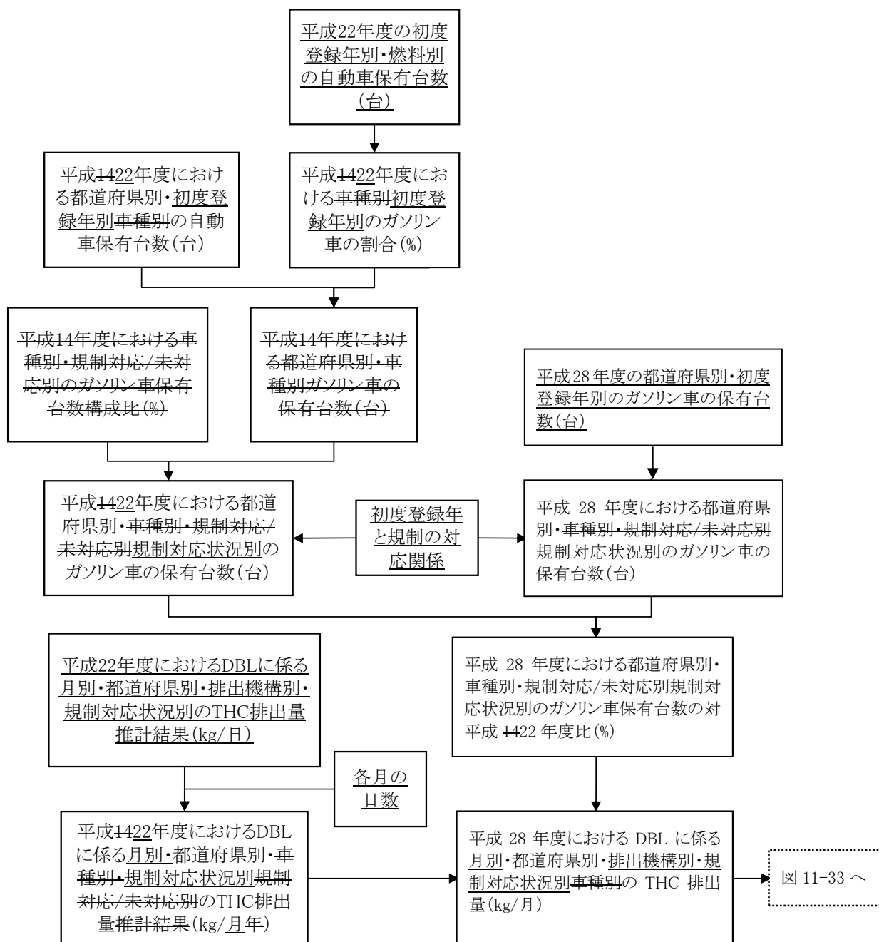
図11-33 DBLに係るTHC排出量の推計フロー
