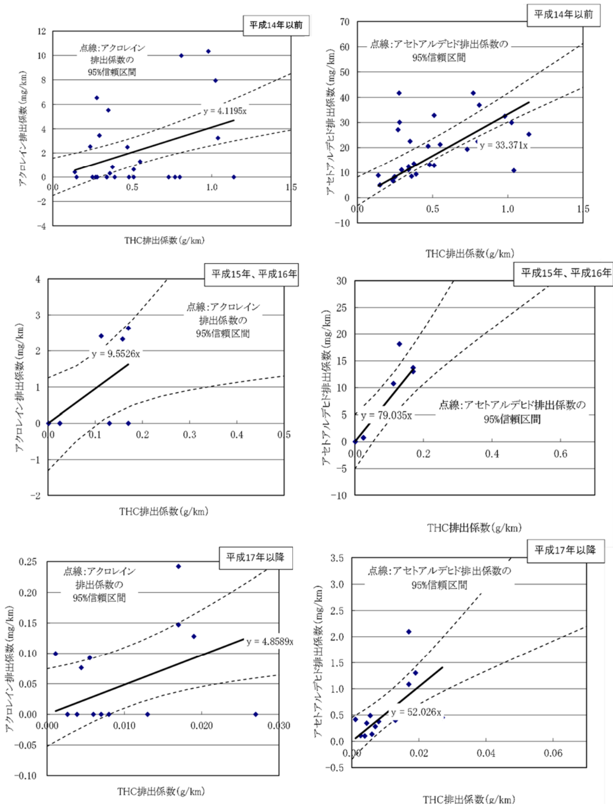
図11-43 ディーゼル自動車(ホットスタート:重量車)に係る THC 排出量と対象化学物質別排出量の比率(その1)
