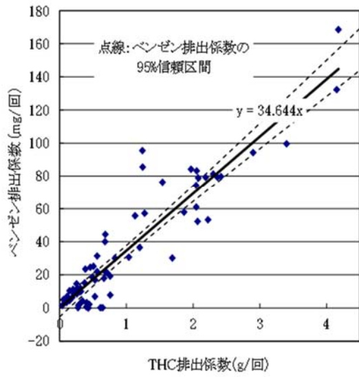
図11-44 ガソリン自動車(コールドスタート時の増分)に係るTHC排出量と対象化学物質別排出量の比率(その3)
