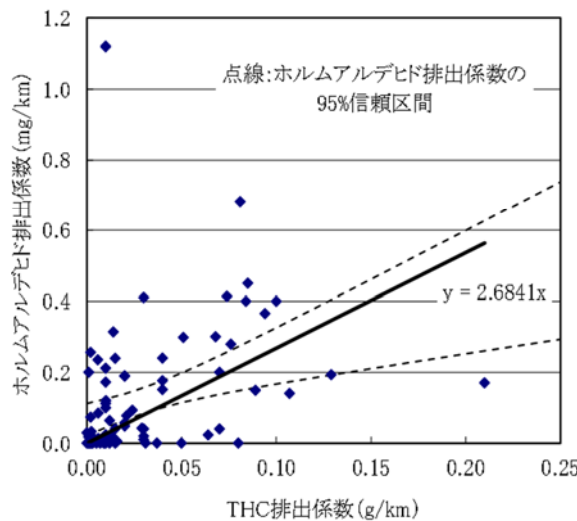
図11-40 ガソリン自動車(ホットスタート)に係る THC 排出量と対象化学物質別排出量の比率(その3)
