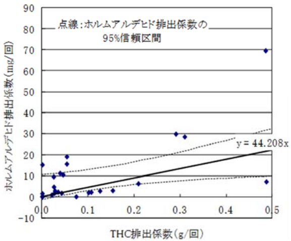
図11-45 ディーゼル自動車(コールドスタート時の増分)に係るTHC排出量と対象化学物質別排出量の比率(その2)
