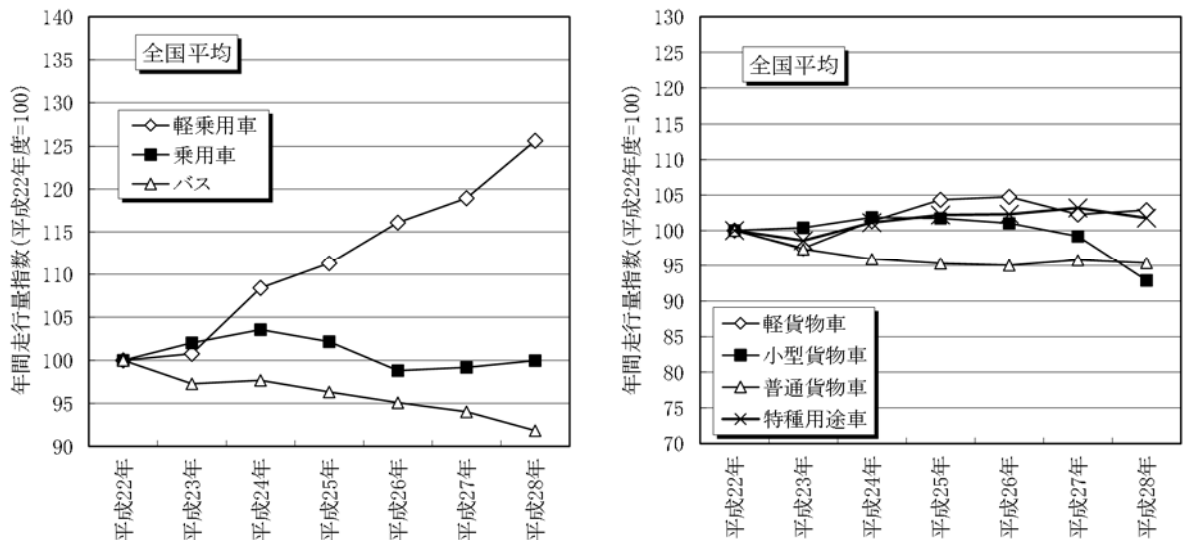
図11-7 全国における車種別年間走行量指数の推移
