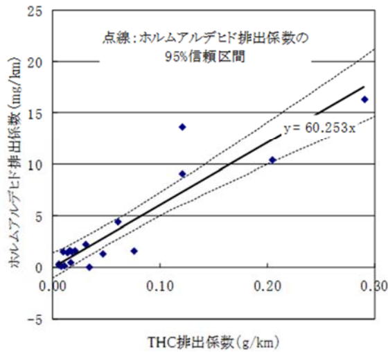
図11-41 ディーゼル自動車(ホットスタート:重量車以外(触媒あり))に係る THC 排出量と対象化学物質別排出量の比率(その2)
