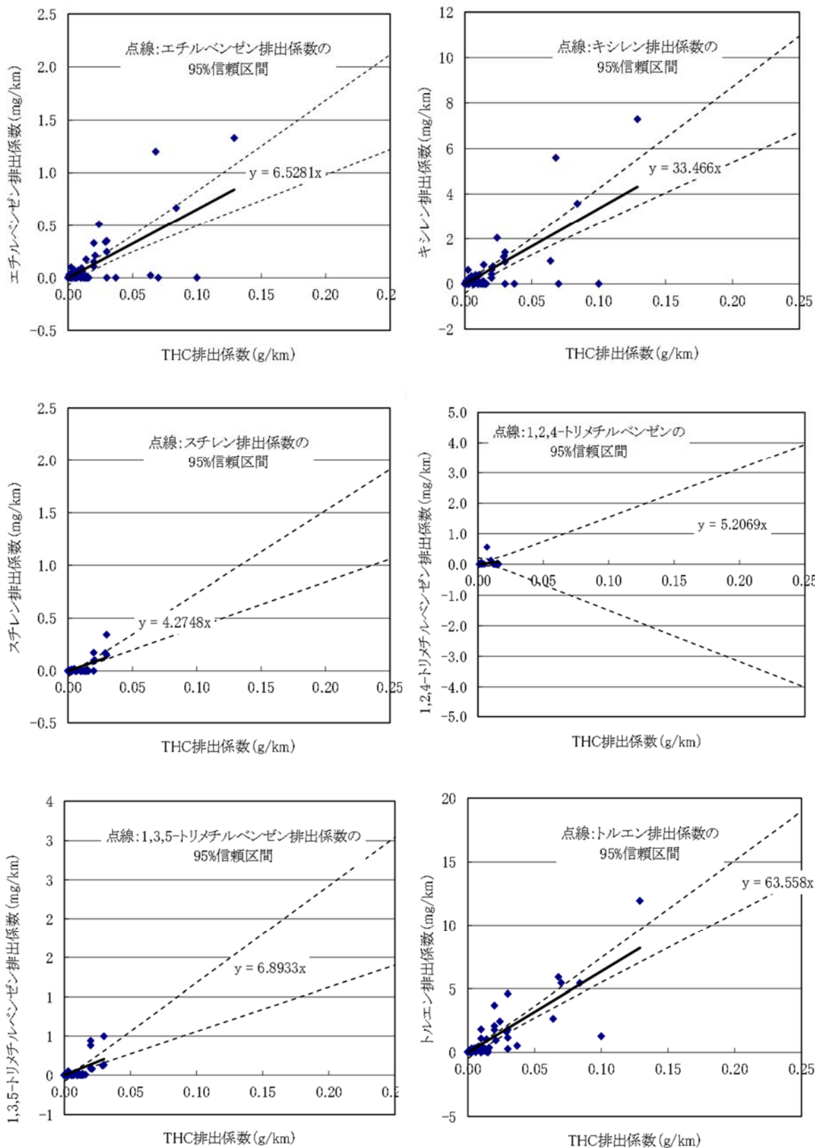
図11-40 ガソリン自動車(ホットスタート)に係る THC 排出量と対象化学物質別排出量の比率(その2)
