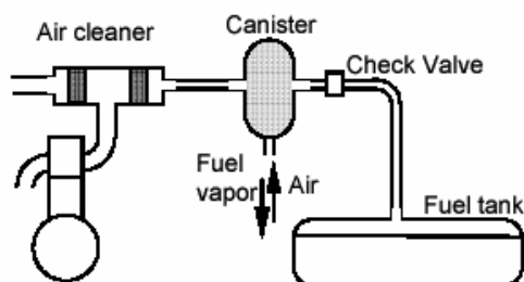
図11-32 燃料タンクとキャニスタの構造
