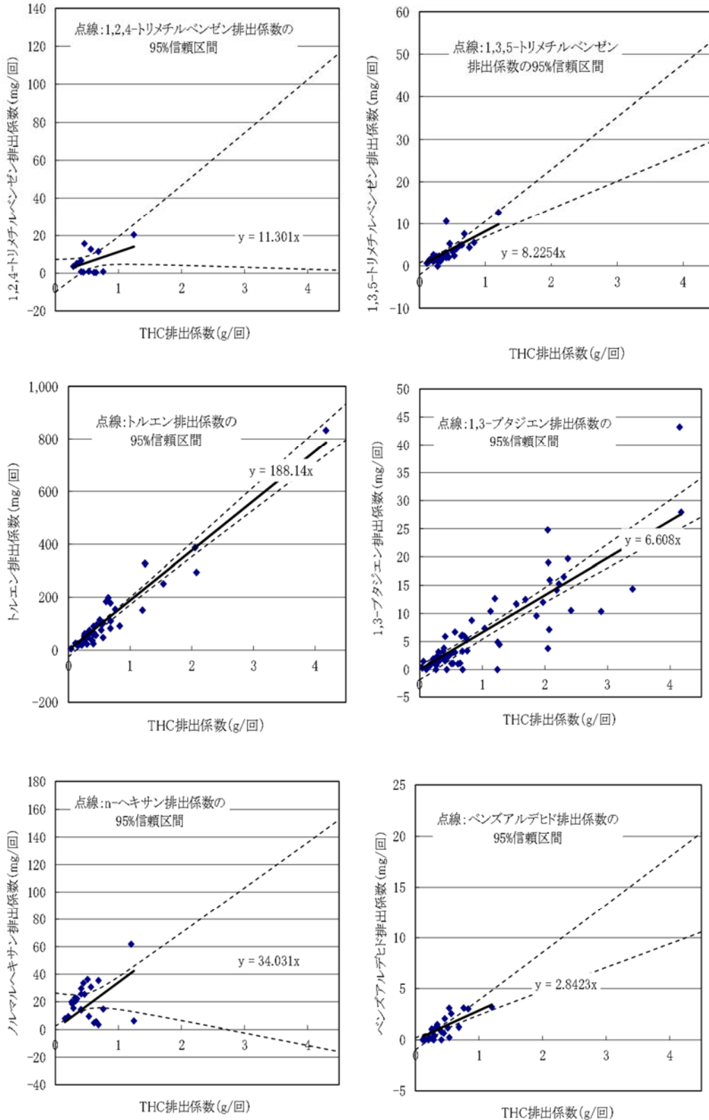
図11-44 ガソリン自動車(コールドスタート時の増分)に係るTHC排出量と対象化学物質別排出量の比率(その2)
