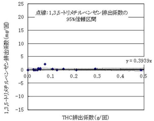
図11-45 ディーゼル自動車(コールドスタート時の増分)に係る THC 排出量と対象化学物質別排出量の比率(その1)
