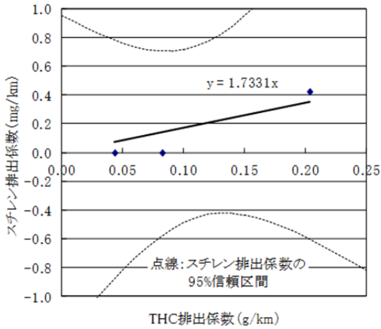
図11-39 ディーゼル自動車(ホットスタート: 重量車以外(触媒なし))に係る THC 排出量と対象化学物質別排出量の比率(その1)
