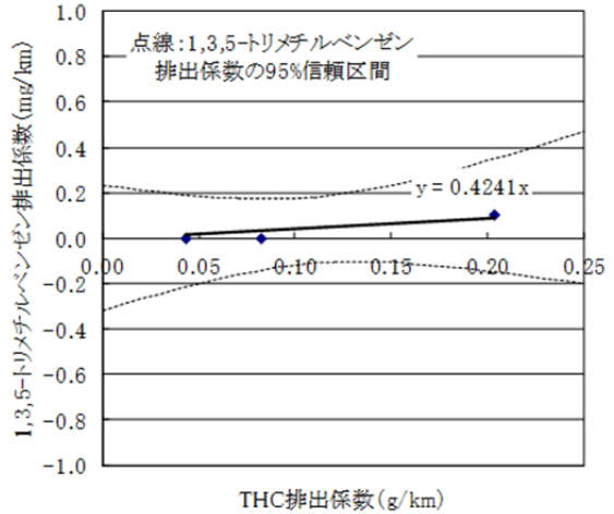
図11-39 ディーゼル自動車(ホットスタート: 重量車以外(触媒なし))に係る THC 排出量と対象化学物質別排出量の比率(その1)
