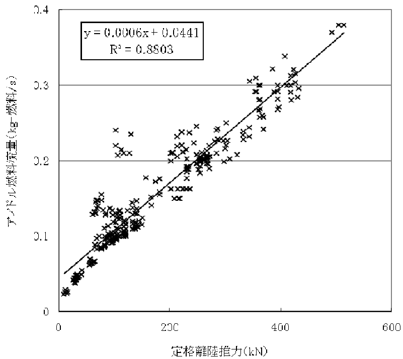
図 16-2 定格離陸推力と燃料流量の関係(アプローチ及びアイドル)
