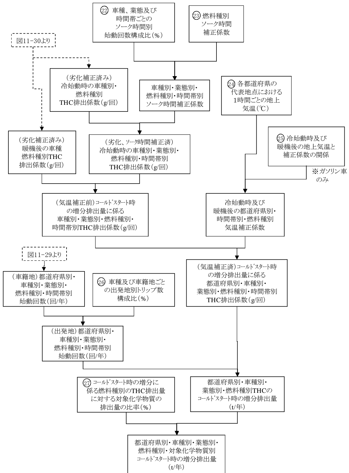
図11-31 都道府県別・車種別・燃料種別対象化学物質排出係数の推計フロー
