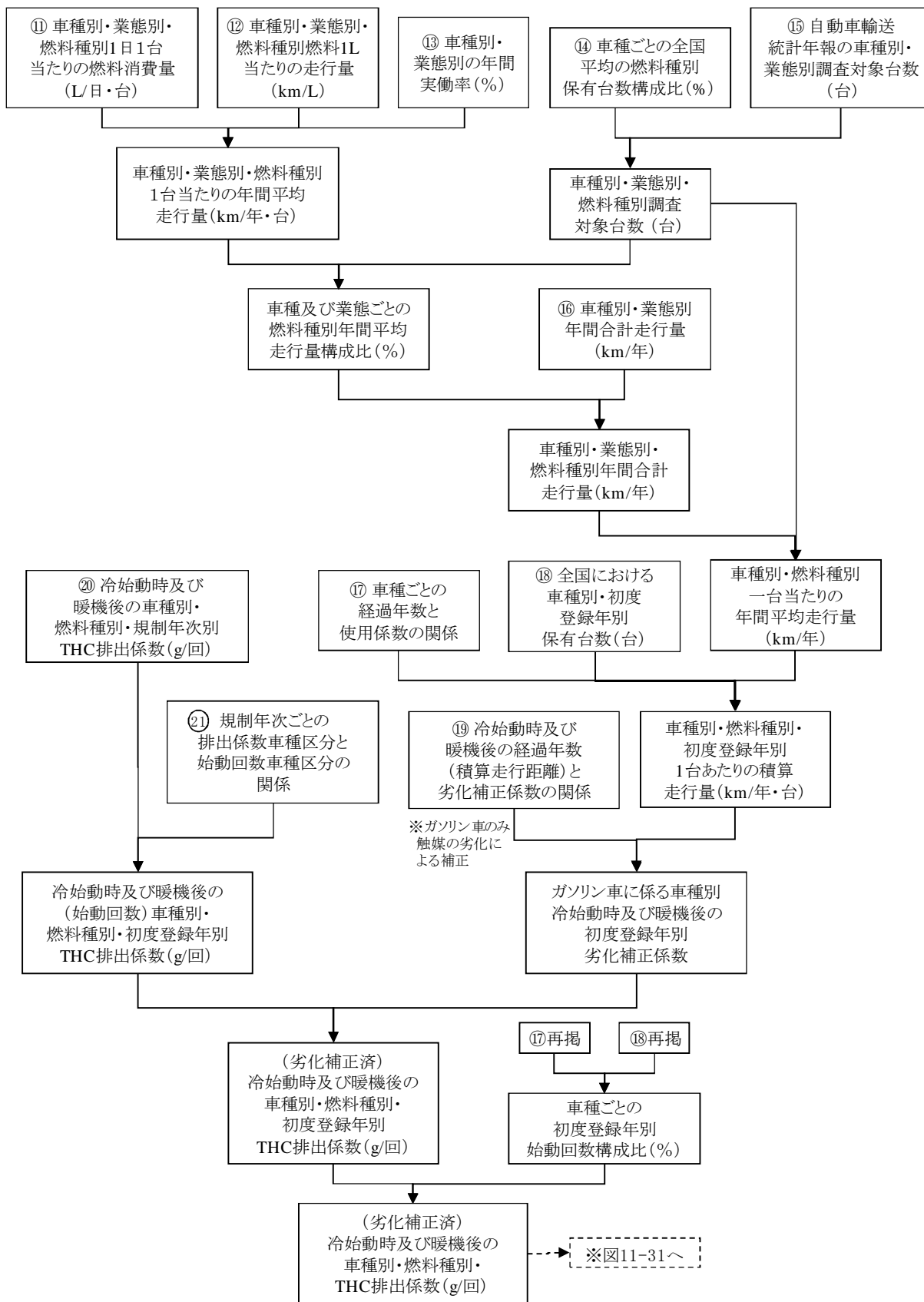
図11-30 劣化補正済車種別・燃料種別 THC 排出係数の推計フロー
