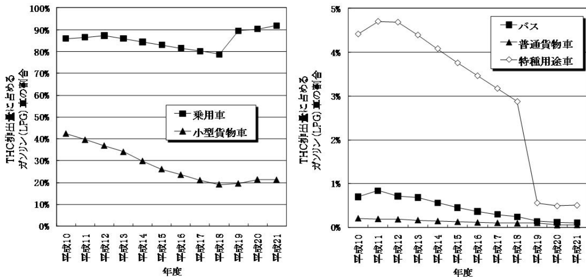
図11-13 自動車排ガスのTHC排出量に占めるガソリン車の割合の推移
