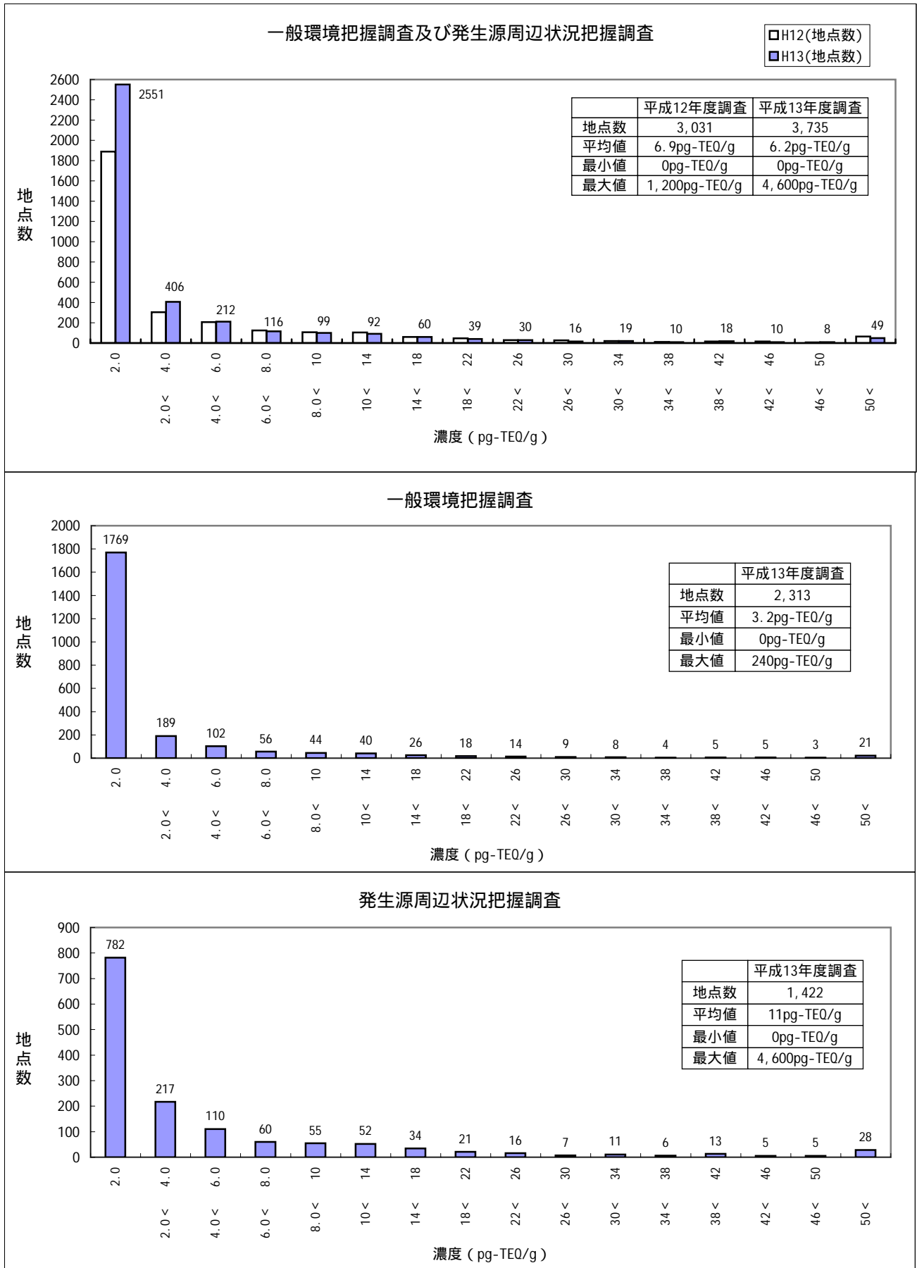
図6 平成13年度ダイオキシン類環境調査結果（土壌）の濃度分布
