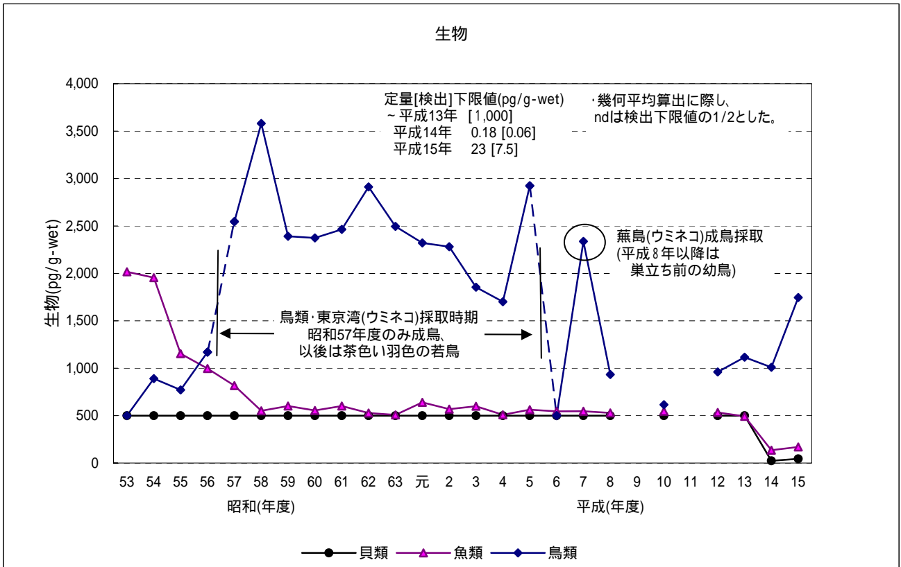
図13 H C Bの経年変化図(幾何平均値)
