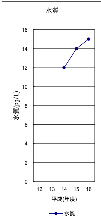
図3-10-A p,p' -DDTの水質の経年変化(幾何平均値)
