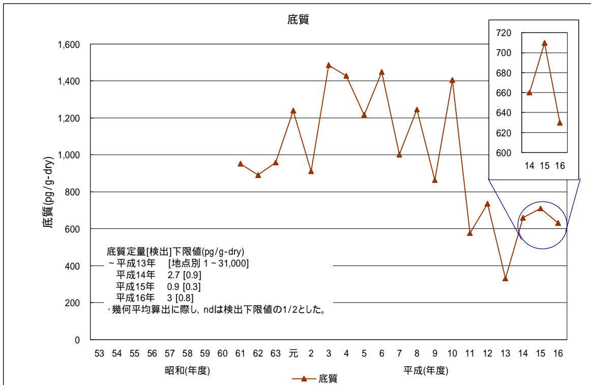
図3-11-B p,p' -DDEの底質の経年変化(幾何平均値)
