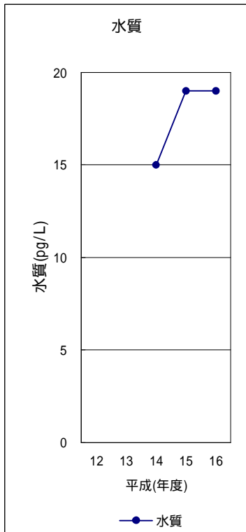
図3-12-A p,p' -D D Dの水質の経年変化(幾何平均値)
