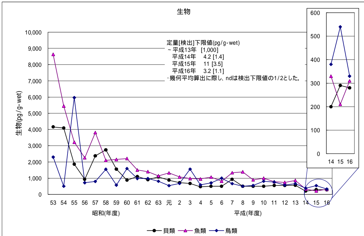
図3-10-C p,p' -DDTの生物の経年変化(幾何平均値)
