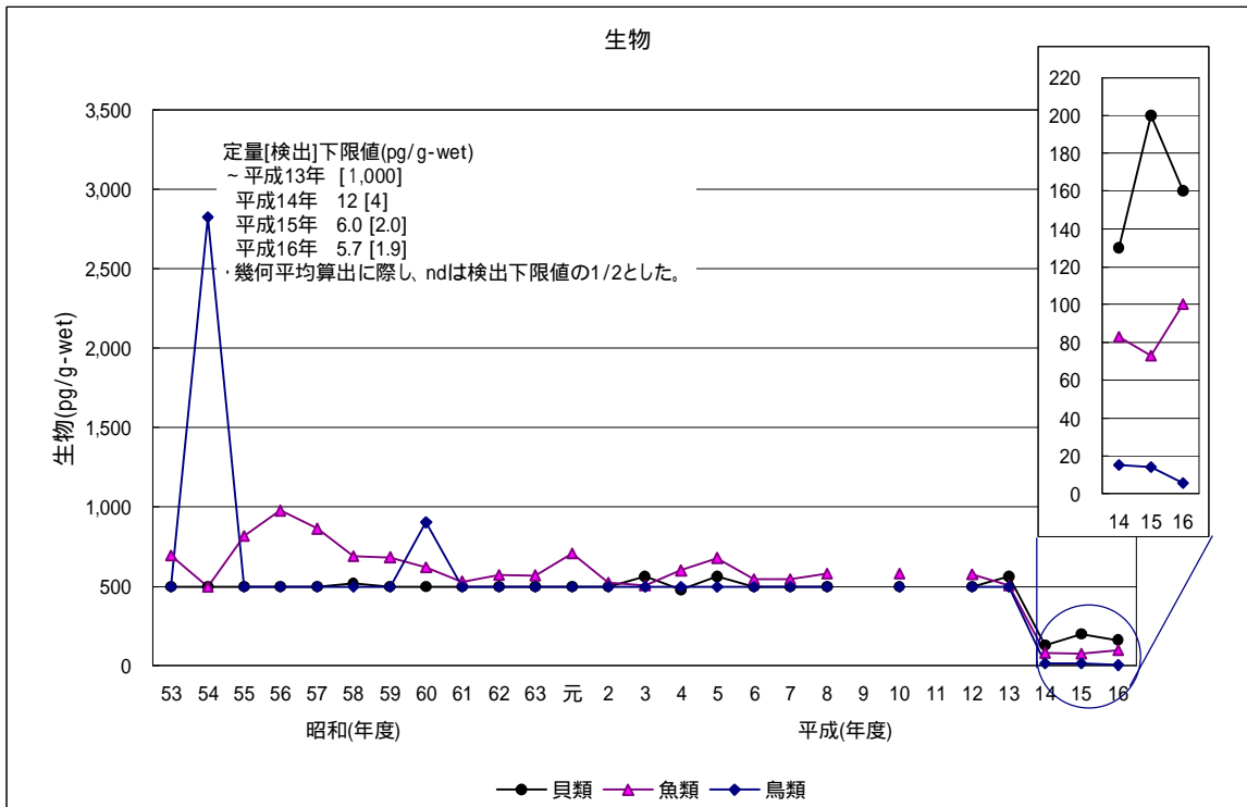
図3-15-C o,p'-DDDの生物の経年変化(幾何平均値)
