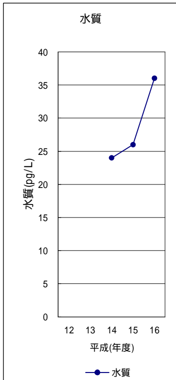
図3-11-A p,p' -DDEの水質の経年変化(幾何平均値)
