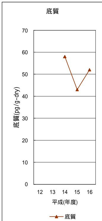
図3-13-A o,p' -DDTの水質の経年変化(幾何平均値)
