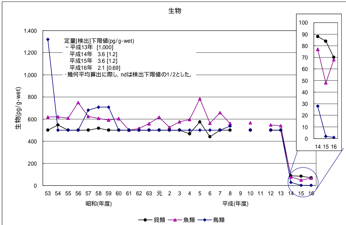
図3-14-C o,p' -DDEの生物の経年変化(幾何平均値)
