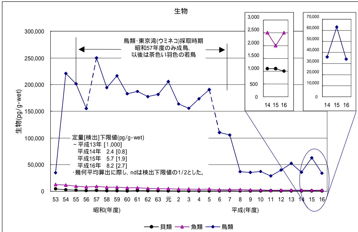
図3-11-C p,p' -DDEの生物の経年変化(幾何平均値)
