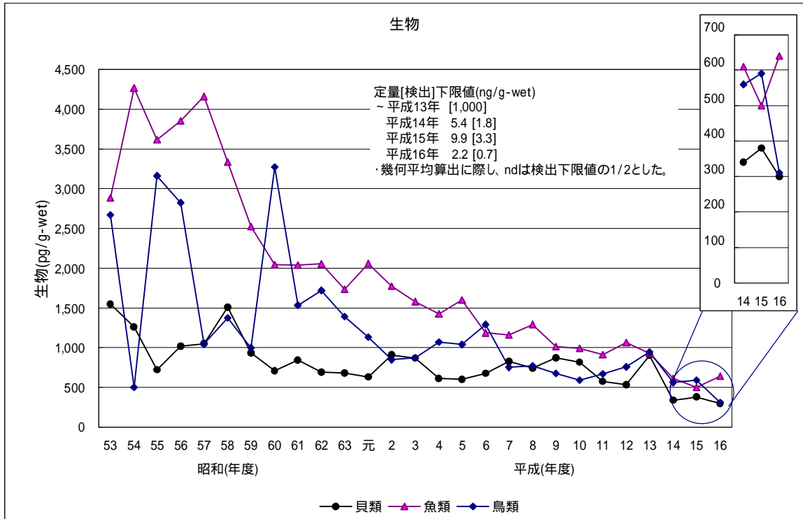
図3-12-C p,p' -DDDの生物の経年変化(幾何平均値)
