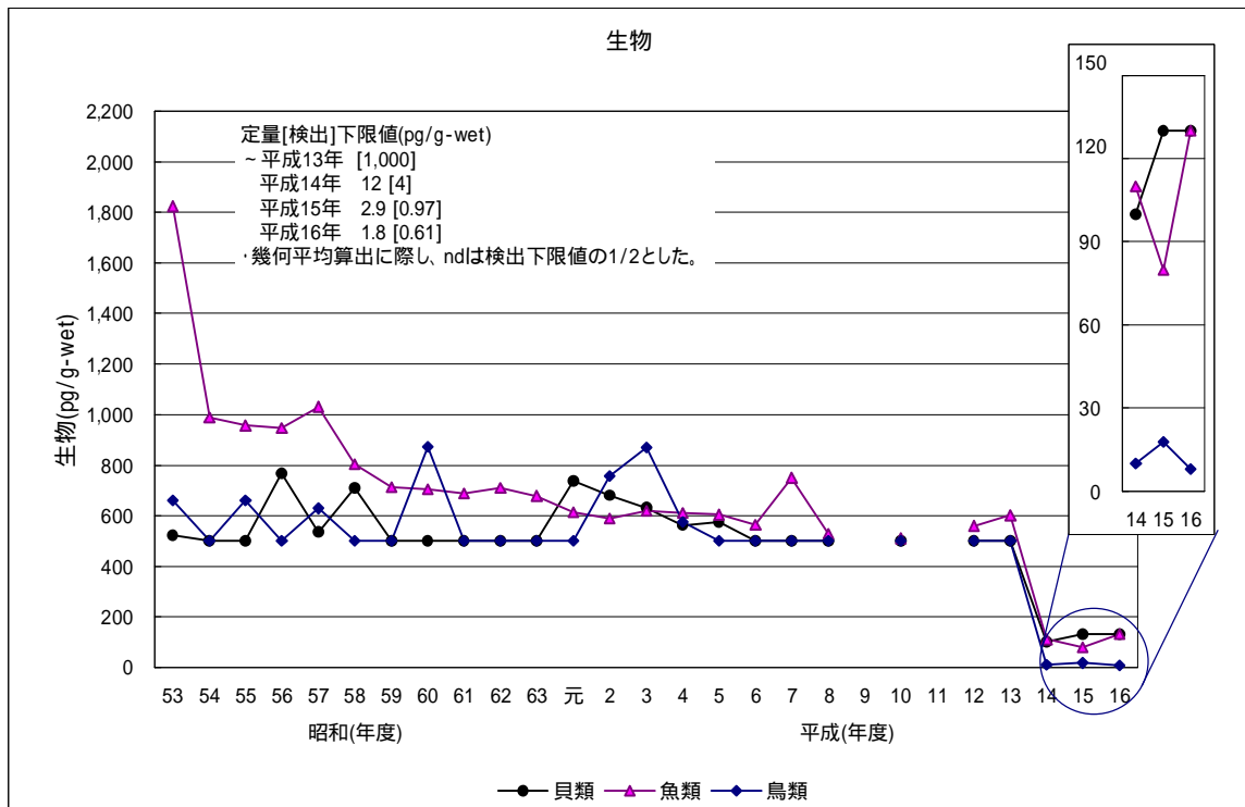
図3-13-C o,p' -DDTの生物の経年変化(幾何平均値)
