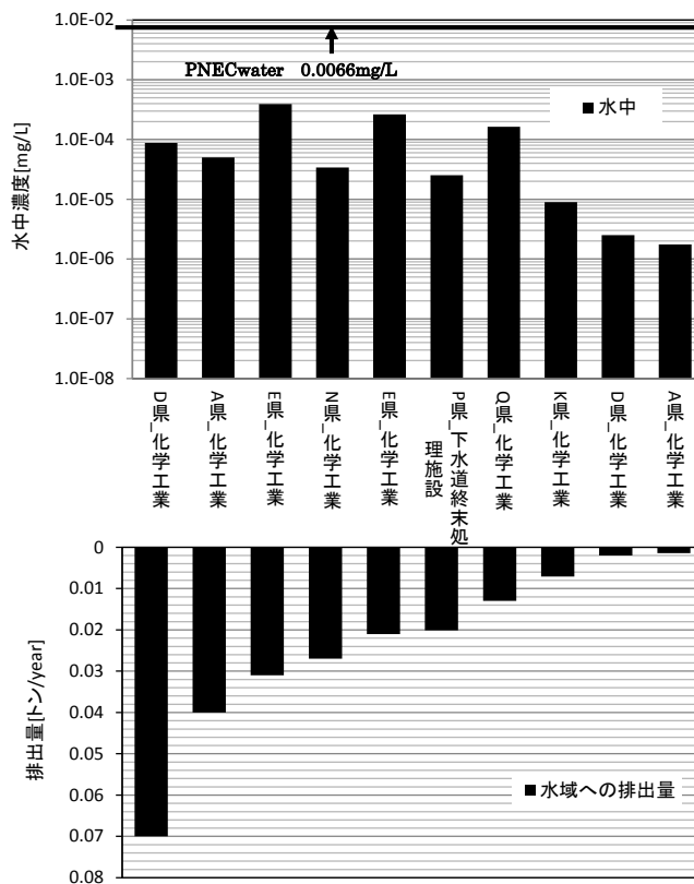
7 8 図 5-5 PRTR 届出事業所毎の排出量に対する水中濃度
