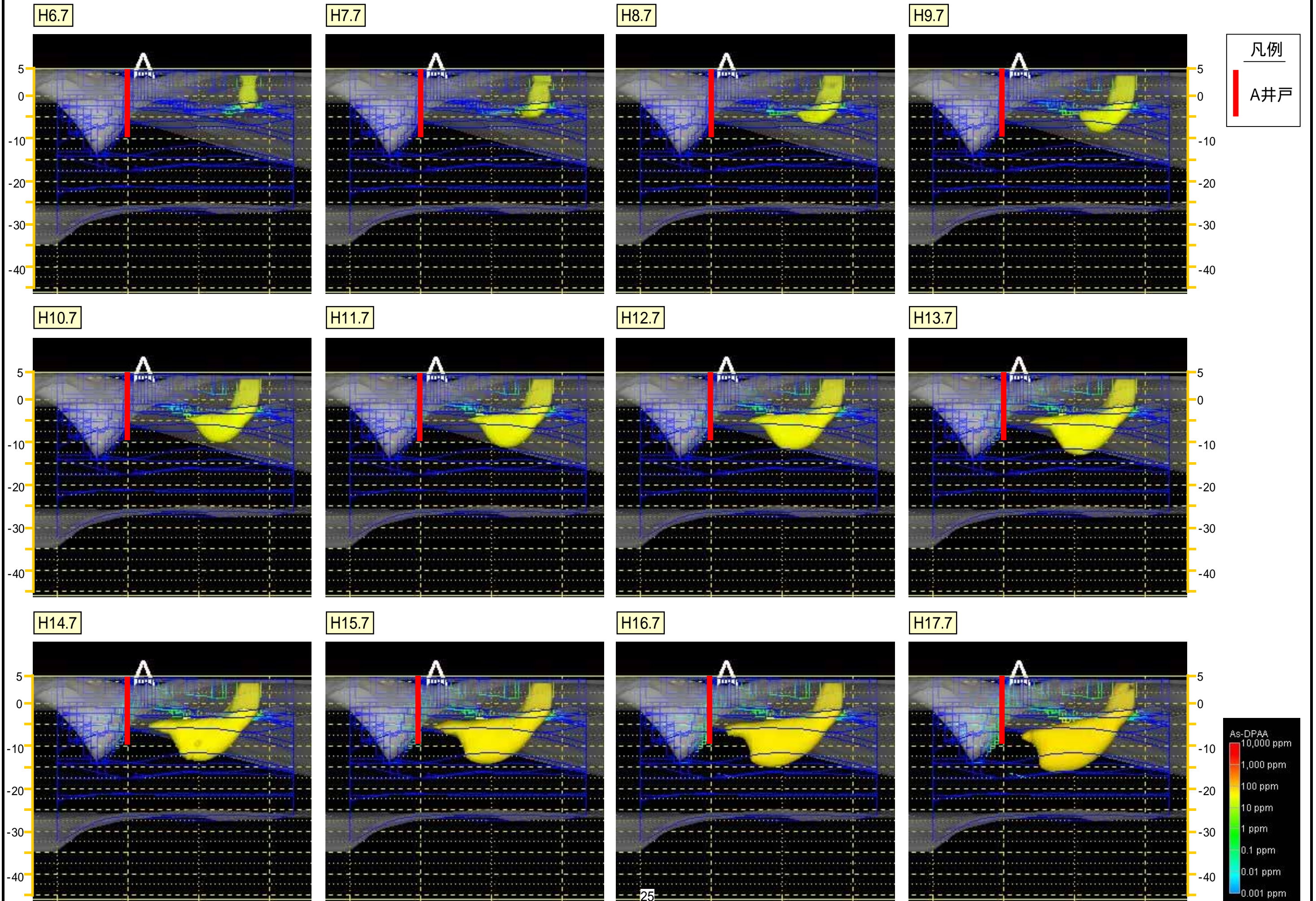
図5.1.4 Case2 初期濃度1,000ppm (ヒ素換算値) 汚染推移 (10ppm)
