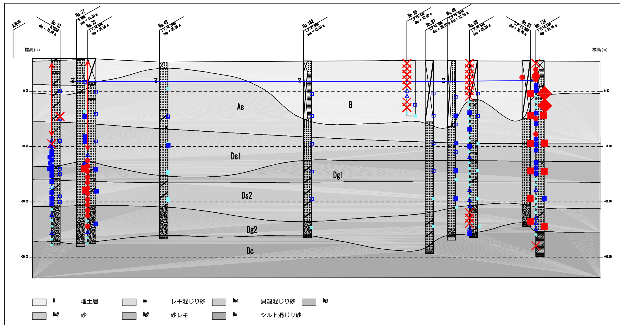
図3.2.2 A井戸から掘削調査地点の地層断面図 (汚染メカニズム中間報告書より)
