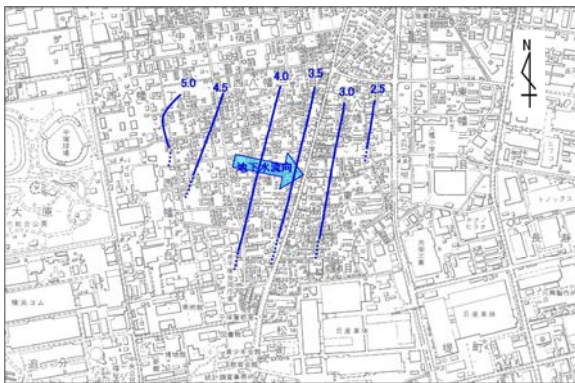
図 1 - 1 地下水の流れと地下水位の等高線 夏季：平成 25 年 9 月測定 (地下水位等高線の単位：標高 m)
