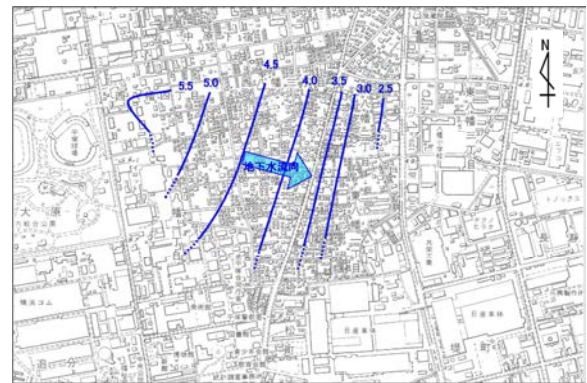
図 1 - 2 地下水の流れと地下水位の等高線 秋季：平成 25 年 11 月測定 (地下水位等高線の単位：標高 m)
