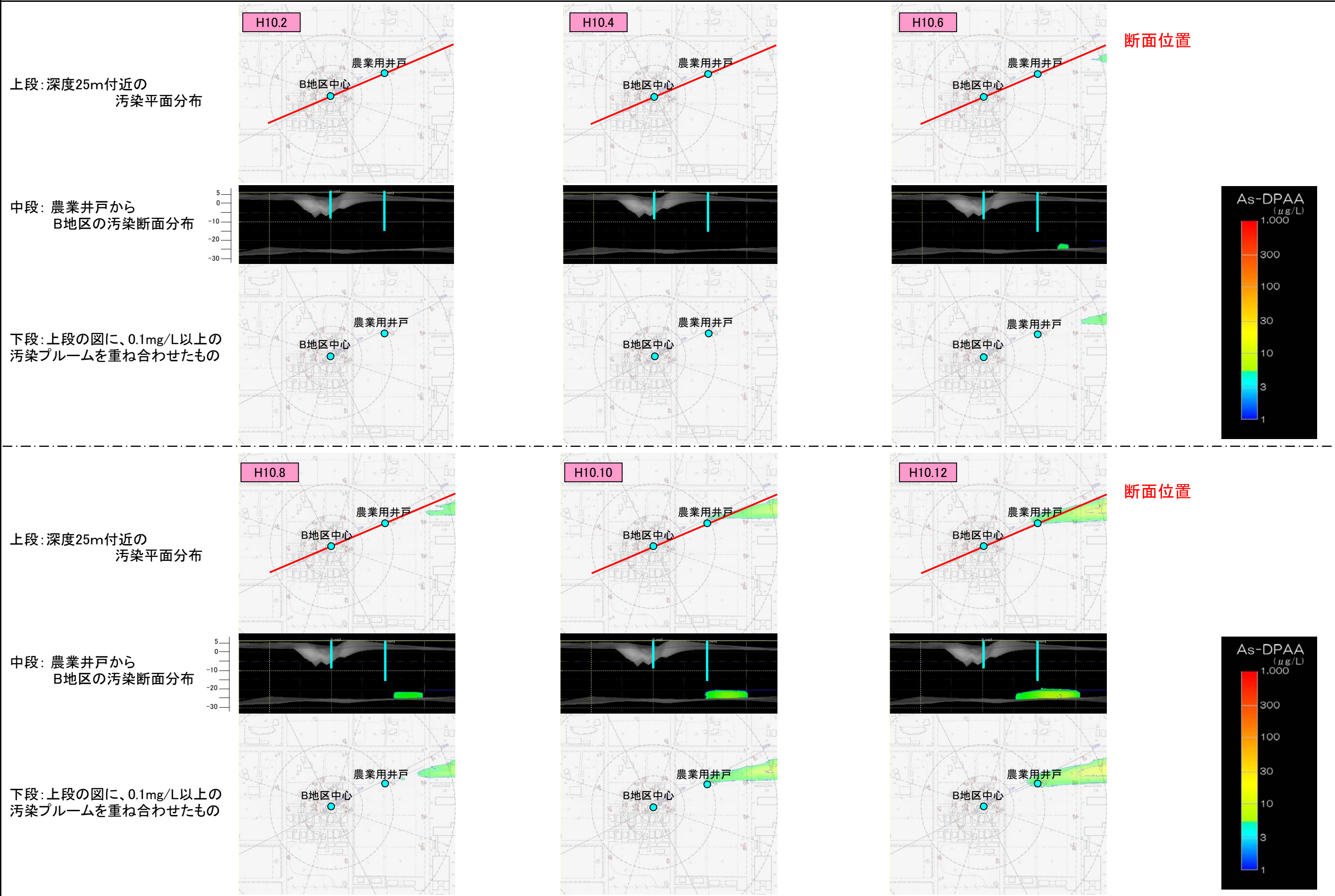
図6.1.4 B地区詳細地下水汚染シミュレーション結果 ①
