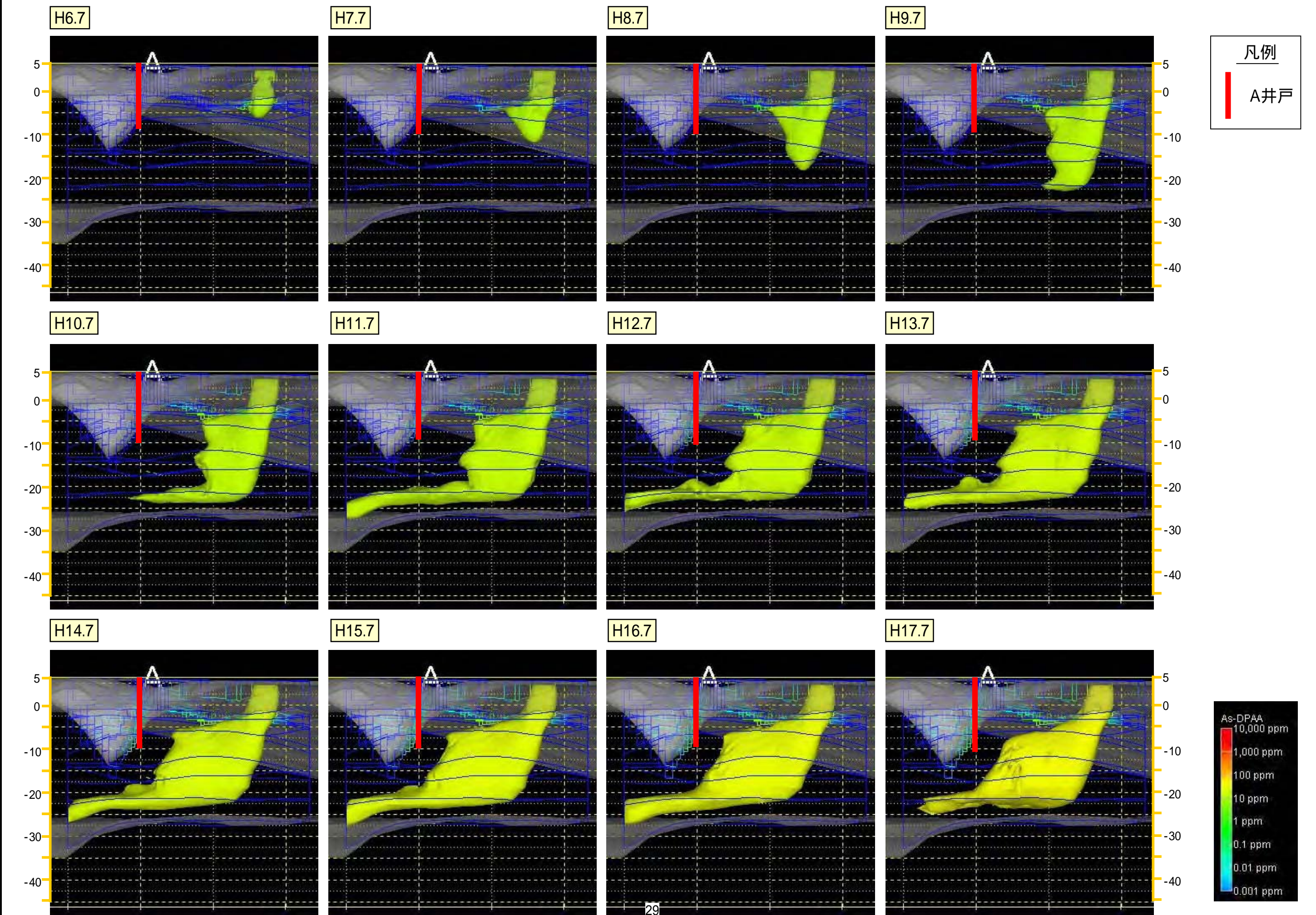
図5.1.6 Case3 初期濃度3,200ppm (ヒ素換算値) 汚染推移 (10ppm)
