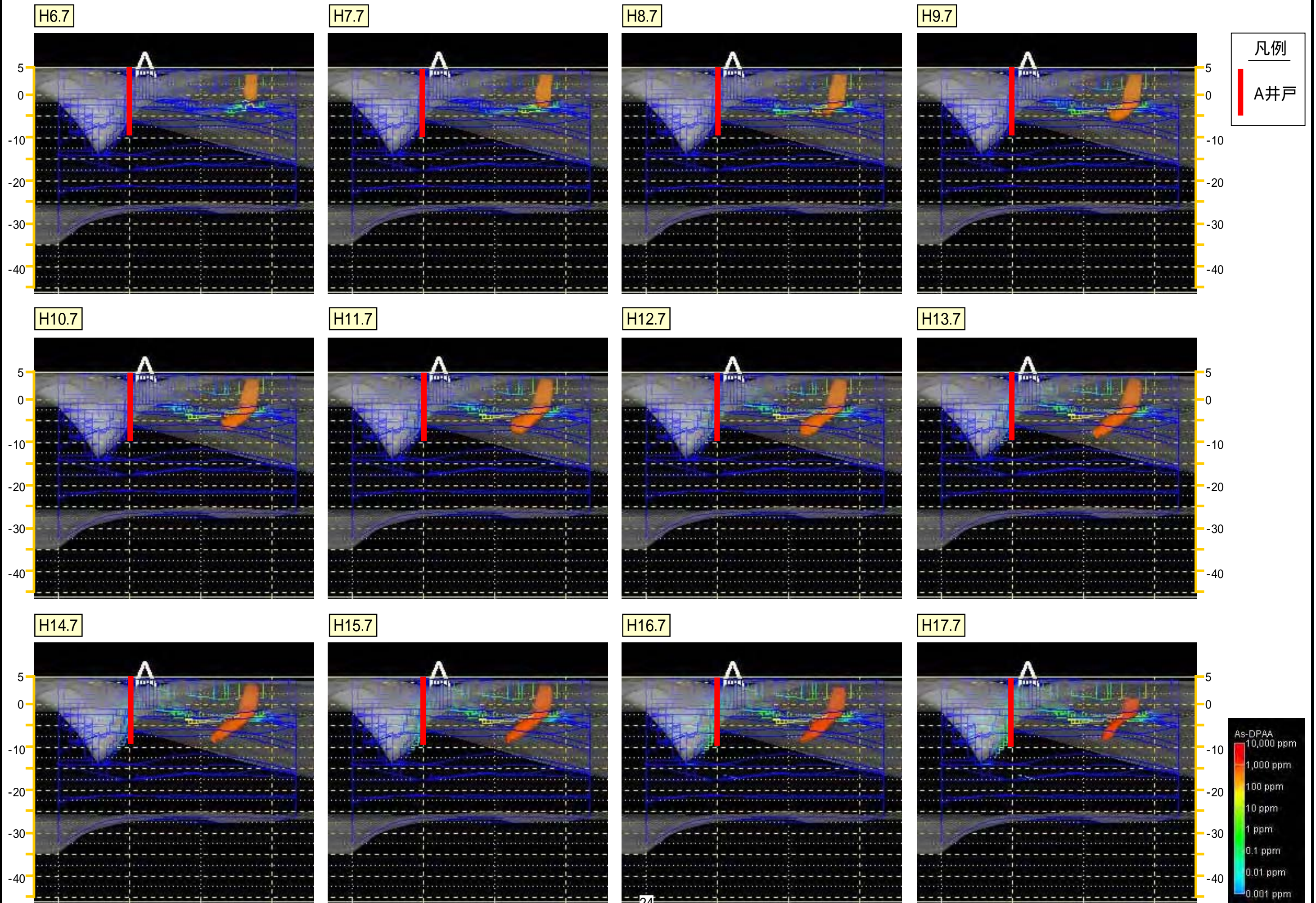
図5.1.4 Case2 初期濃度1,000ppm (ヒ素換算値) 汚染推移 (100ppm)
