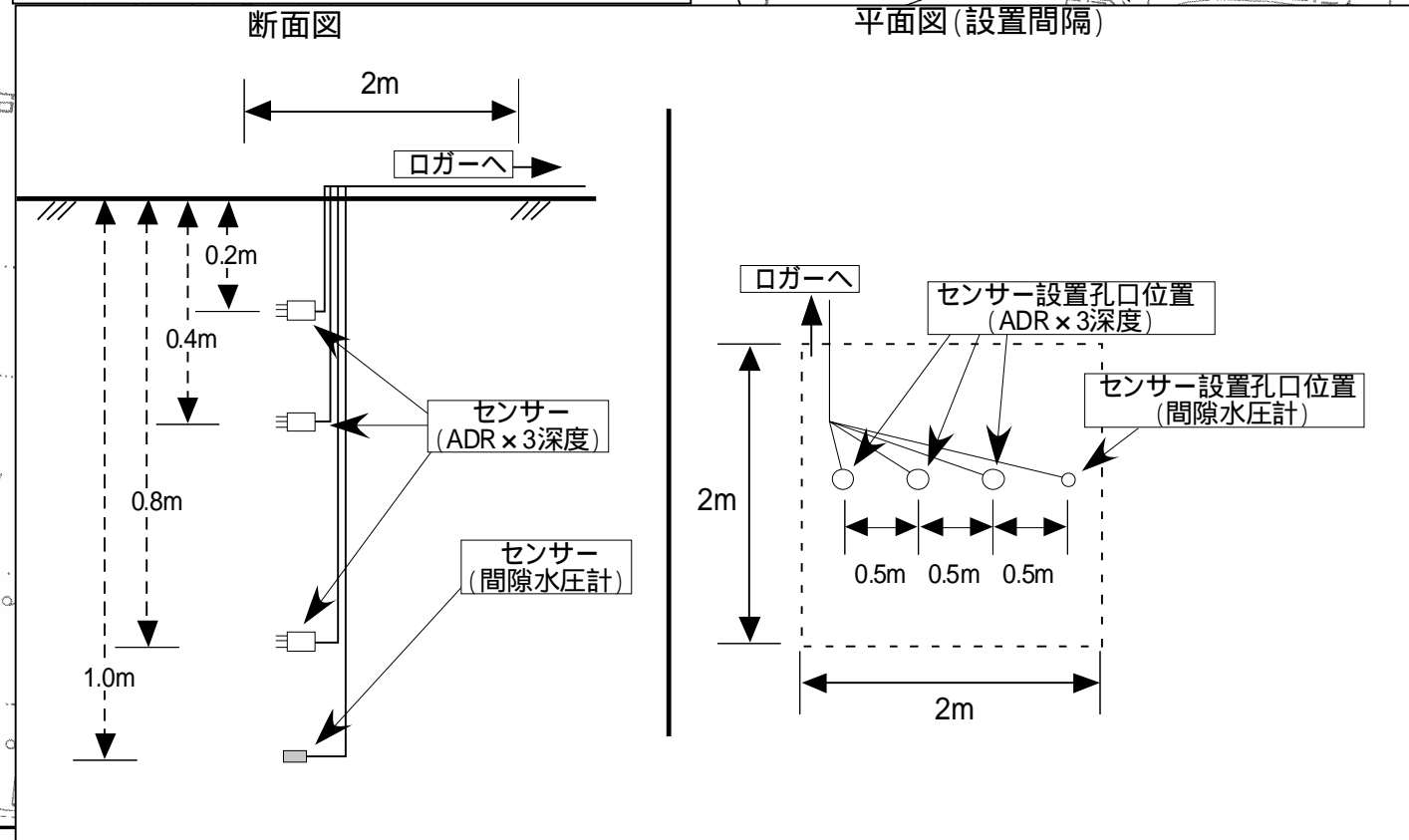
土壌水分計および間隙水圧計設置概念図
