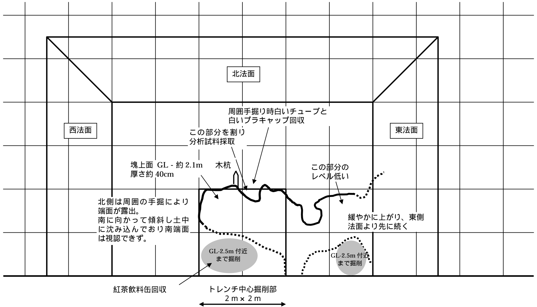
T 5 ( G L 2.0 ~ - 2.5 m ) 大塊物の概略図
