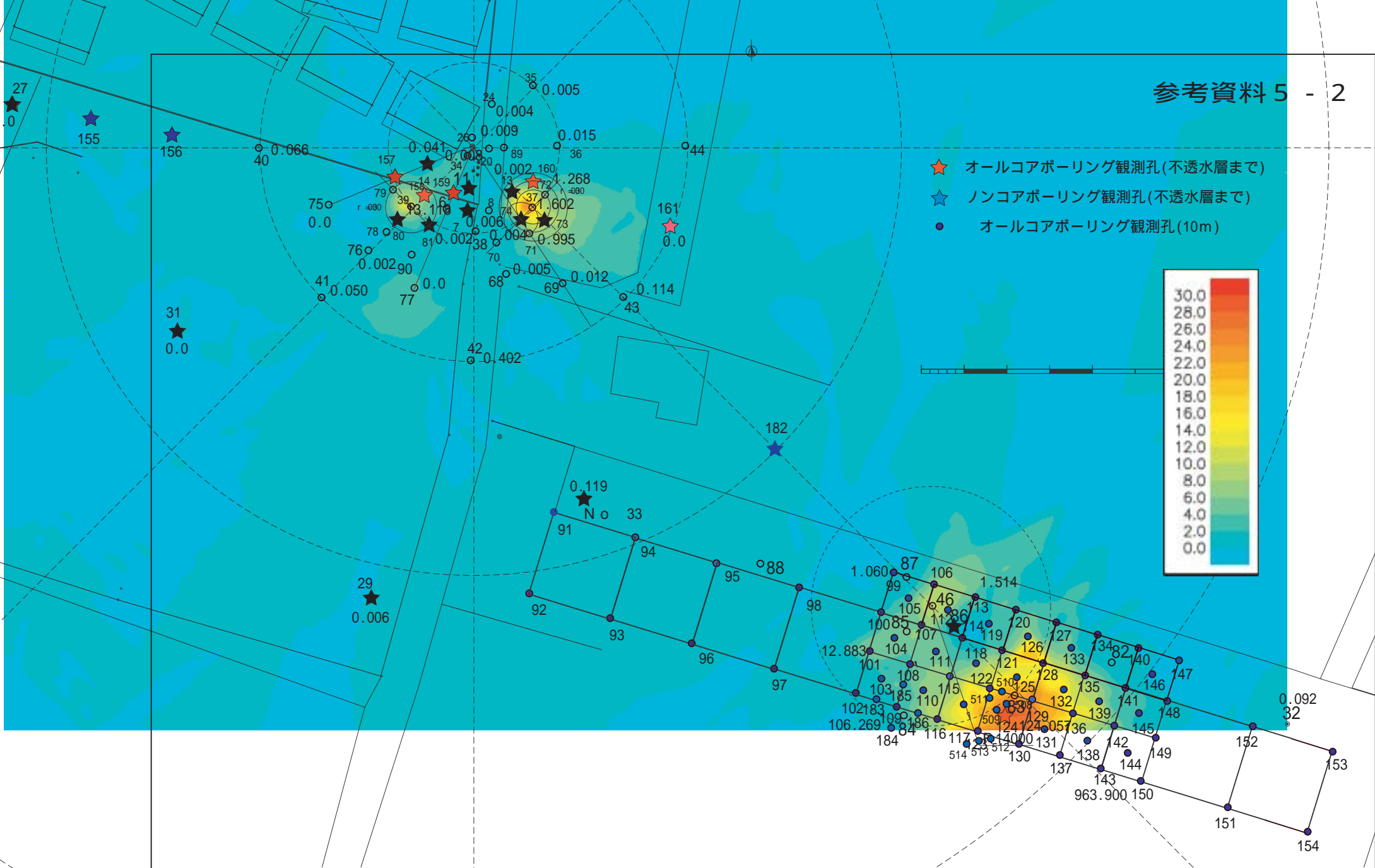
A地区における地下水総ヒ素濃度分布区図(G L -20m)
