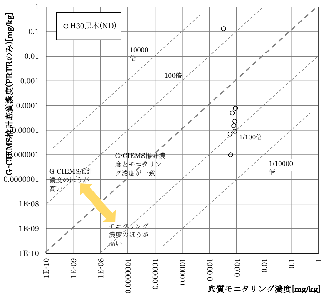
1 2 図 6 G-CIEMS 推計底質濃度(PRTR のみ、平成 28 年度)と底質モニタリング濃度(黒本調査平成 30 3 年度)の比較
