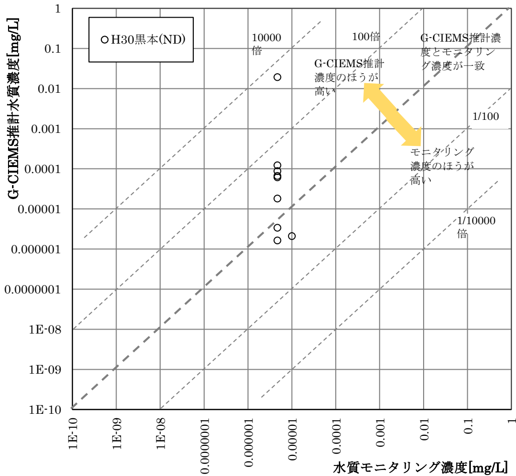
図 3 G-CIEMS 推計水質濃度 (PRTR 及び化審法長期使用用途排出量、平成 28 年度) と水質モニタリング濃度 (黒本調査平成 30 年度) の比較
