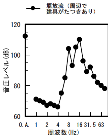
図7.1 堰放流時に発生する低周波音の事例；音源側
