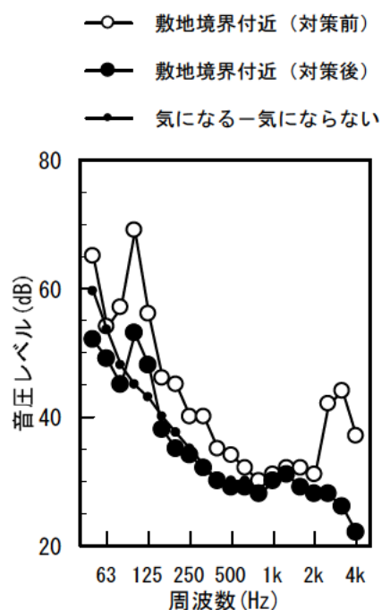
図7.5 低周波音と騒音が複合した「低周波音苦情」の例 ; 家庭用ボイラー
