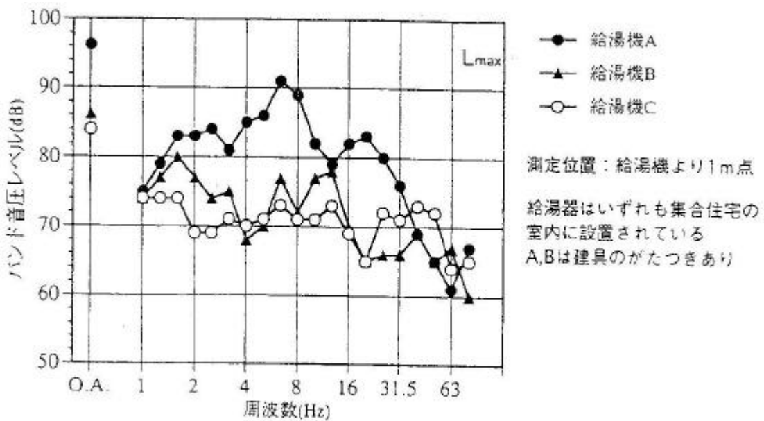
図-e.10 低周波音の周波数特性の例（家庭用ガス給湯暖房機ボイラー）
