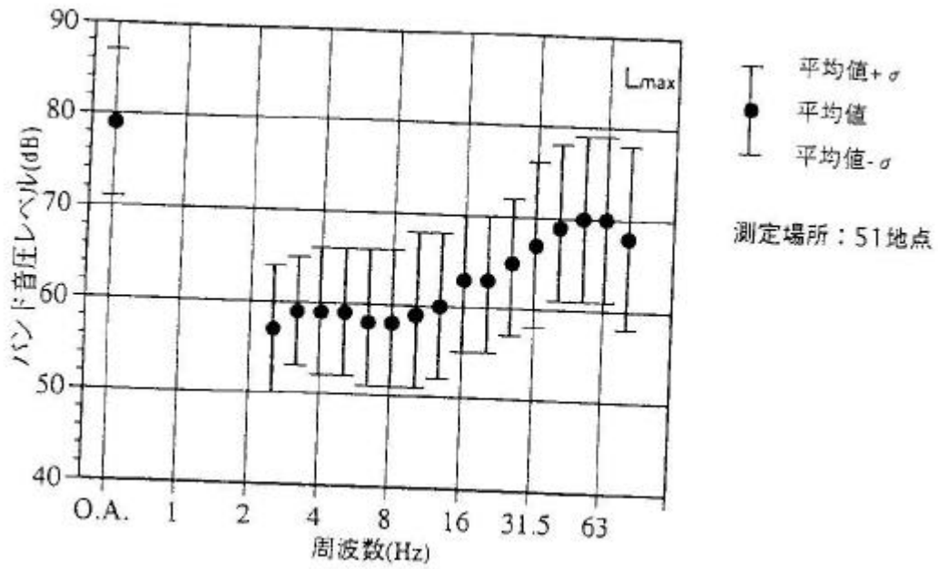
図-e.11 市街地における低周波音の周波数特性の例（商業系地域）
