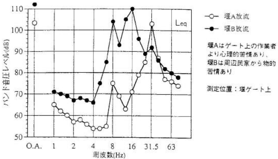
図-e.9 低周波音の周波数特性の例（堰放流）
