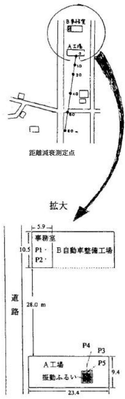
図-5.1.10 室内の音圧分布測定例 (振動ふるい)
