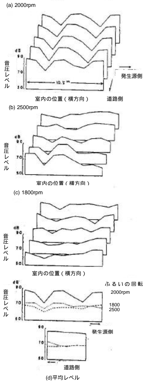
図-5.1.10 室内の音圧分布測定例 (振動ふるい)
