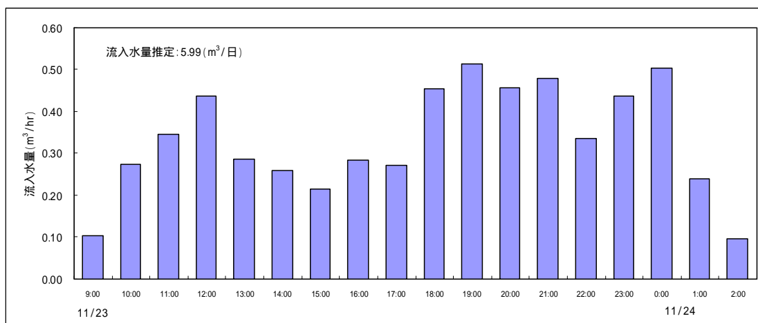
図5 - 1 流入水量の日間変化
