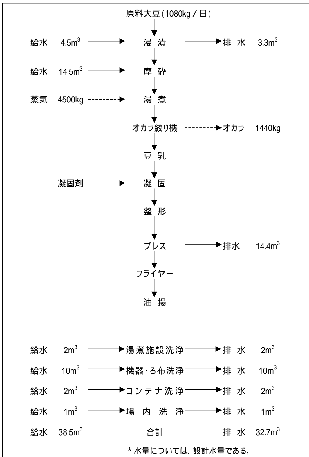
図3 - 1 排水系統図
