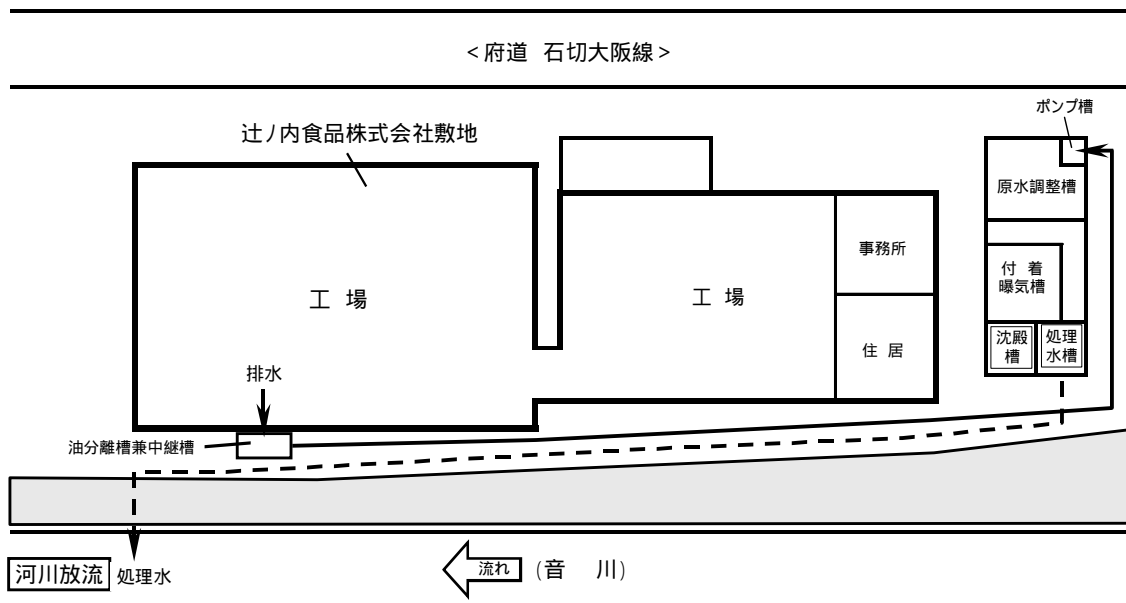
図3 - 2 平面図
