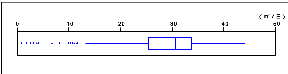
図 5 - 6 流量箱型図
