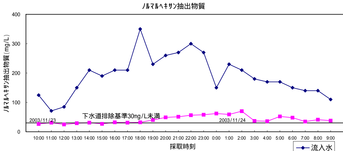
図4 - 1 水質実証項目の日間変化(2) (日間変動の測定 第1回目:平成15年11月23日~24日)
