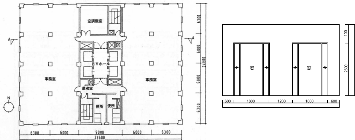
図 2 基準階の平面図（左図）及び立面図（右図）
