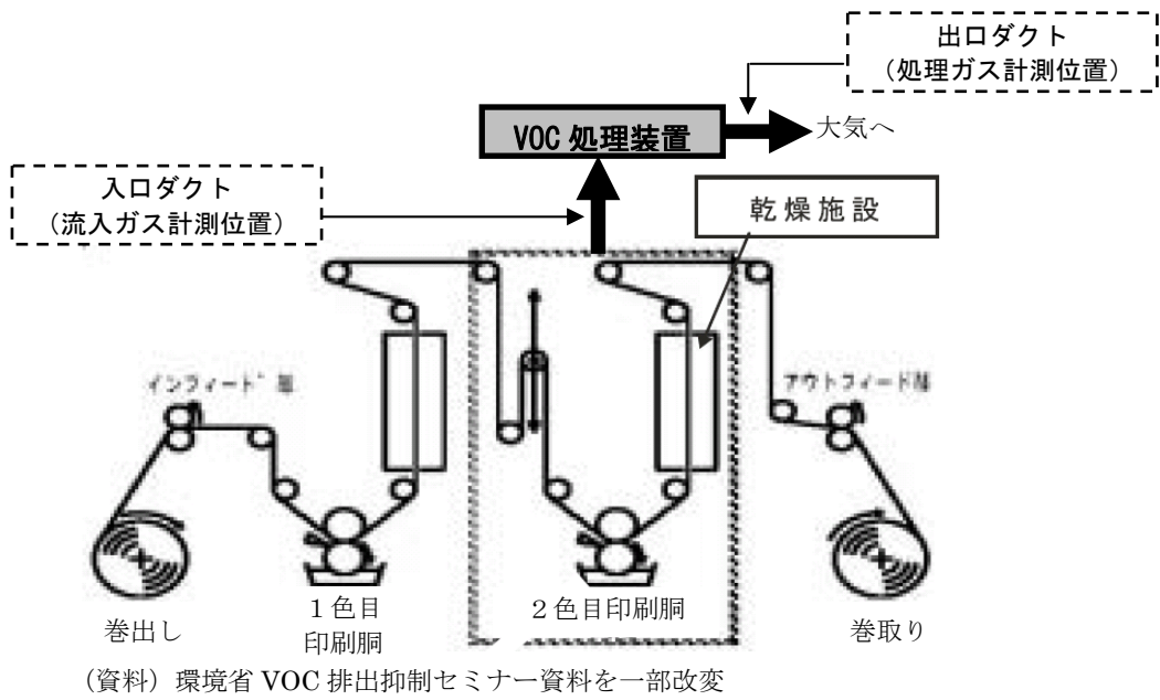
図 3 印刷業における VOC 排出イメージ
