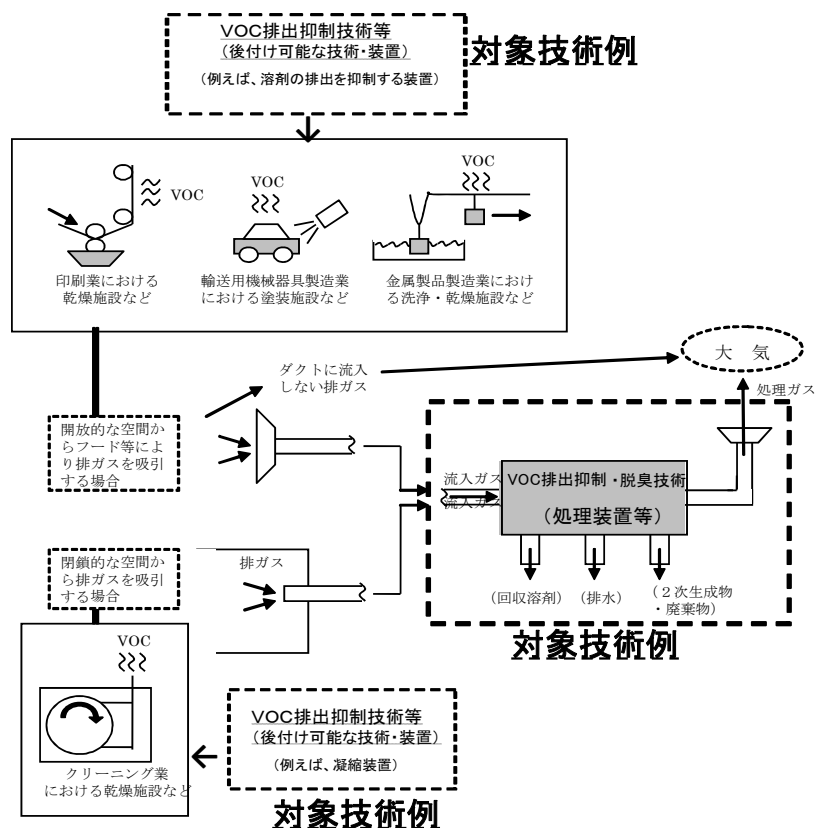
図 1 対象技術のイメージ (点線内が実証対象装置機器)
