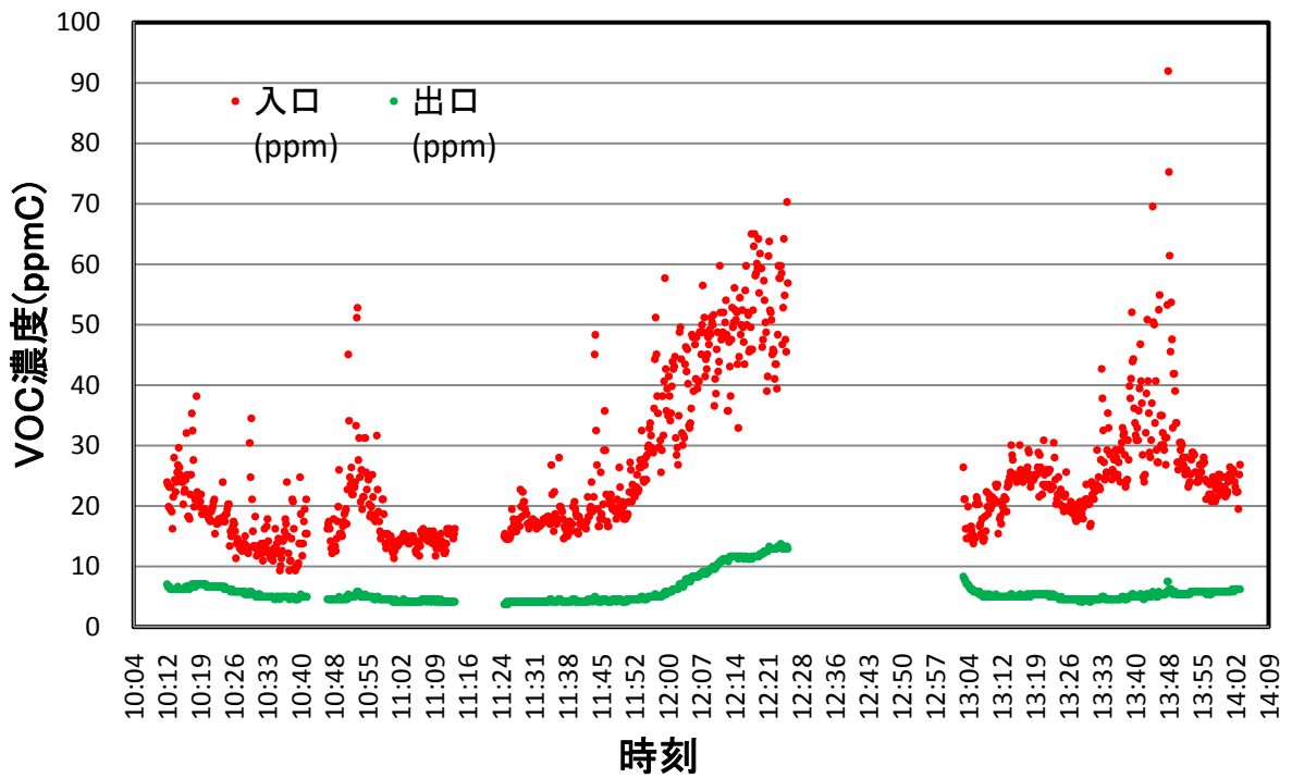
圖 6-8 TVOC 濃度測定結果 (2008/01/24 10 時 12 分~14 時 03 分)
