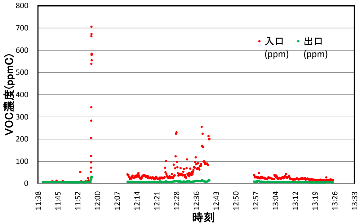
圖 6-7 TVOC 濃度測定結果 (2008/01/22 11 時 40 分~13 時 25 分)
