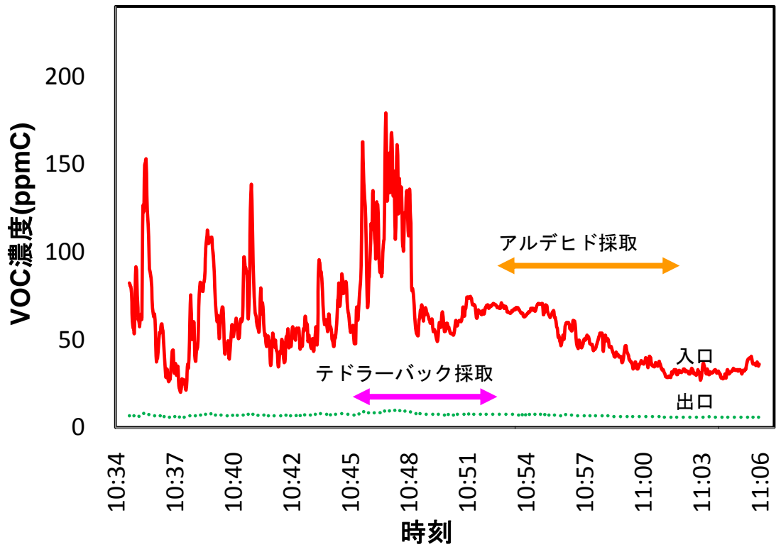
図 6-5 TVOC 濃度測定結果 (2008/01/25 10 時 35 分～11 時 05 分)
