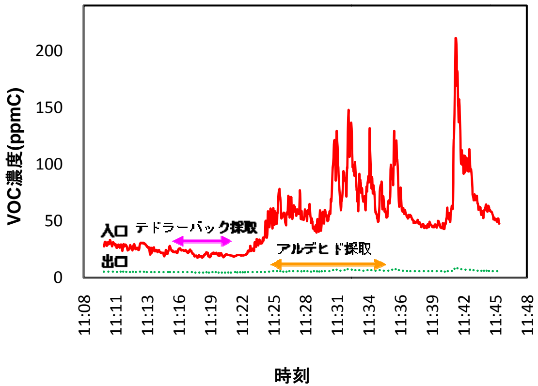
図 6-6 TVOC 濃度測定結果 (2008/01/25 11 時 10 分～11 時 45 分)
