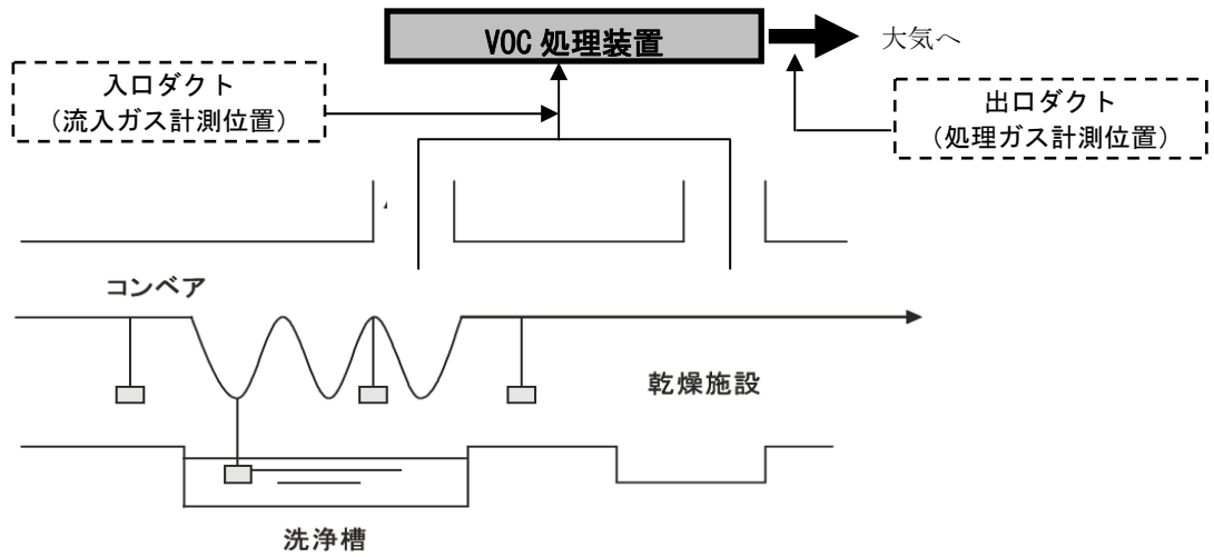
図 4 金属製品製造業における VOC 排出イメージ
