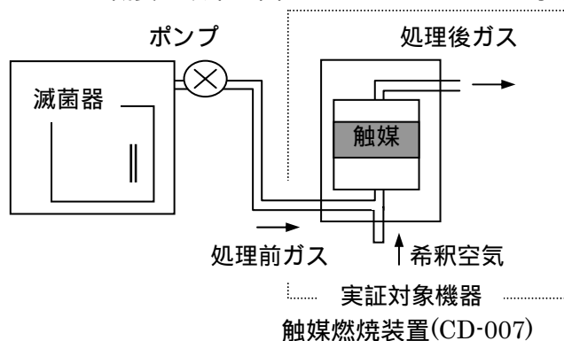
図 3 - 1 : システム概要 (ドライポンプ時)
