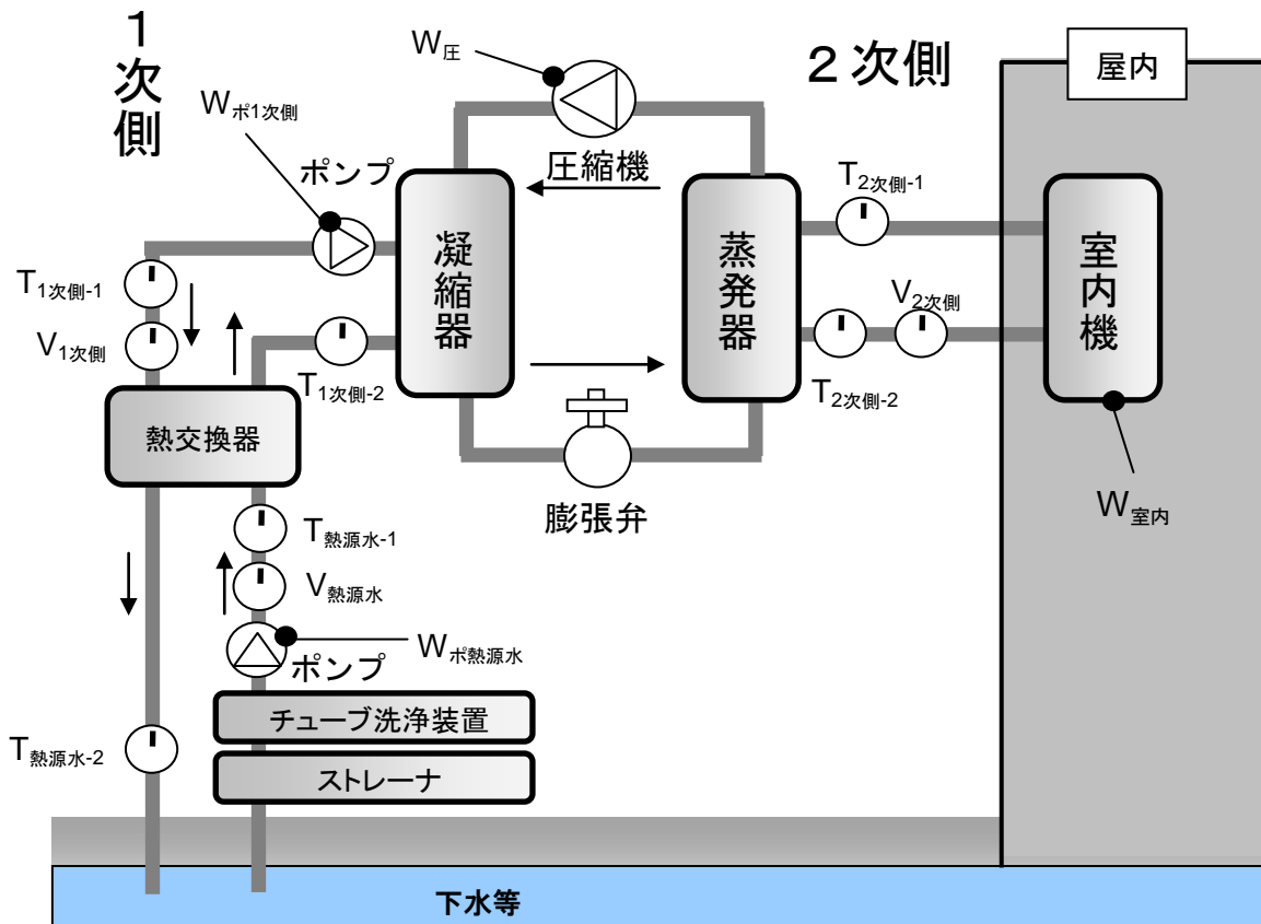
図 6 システム全体の検証における測定箇所 (下水等熱源の場合)
