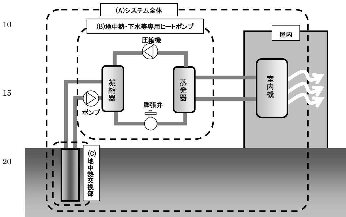
図 2 地中熱・下水等を利用したヒートポンプ空調システム 4
