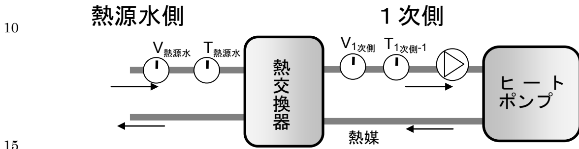
図 10 交換器における測定点
