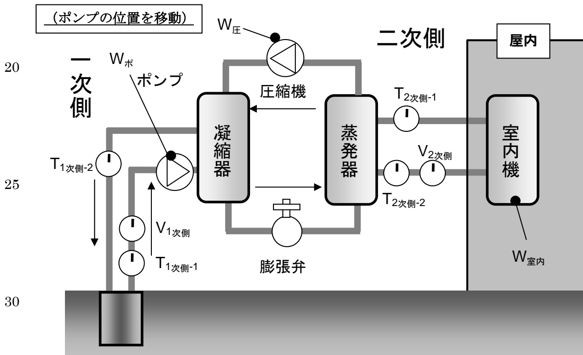
図 4 システム全体の実証における測定箇所 (間接式の場合)
