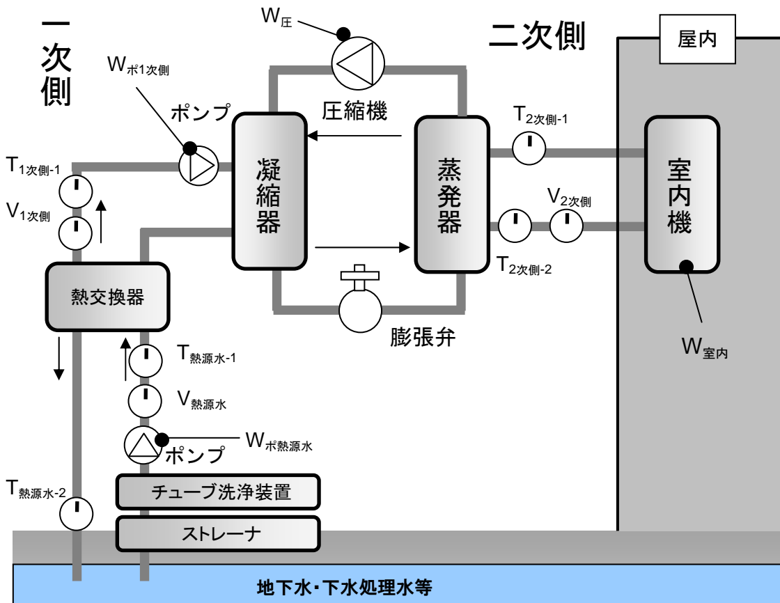
図 6 システム全体の実証における測定箇所 (下水熱源の場合)
