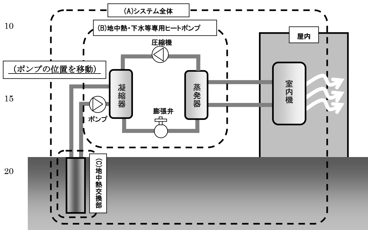
25 図 2 地中熱・下水等を利用したヒートポンプ空調システム 3
