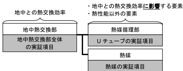
図 8 地中熱交換部における実証項目の構成（熱媒循環式×熱交換器なし）
