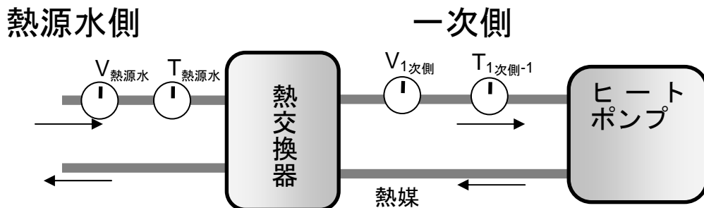
図 10 交換器の熱交換効率の測定における測定点
