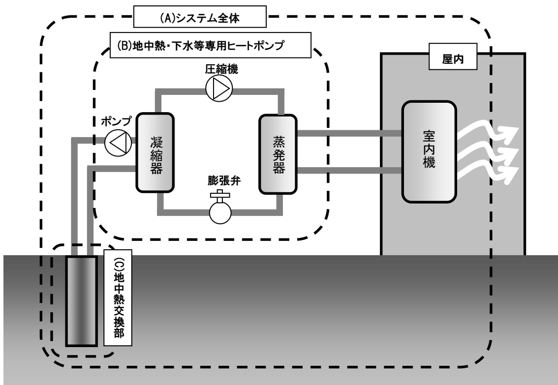
図2 地中熱・下水等を利用したヒートポンプ空調システム 2
