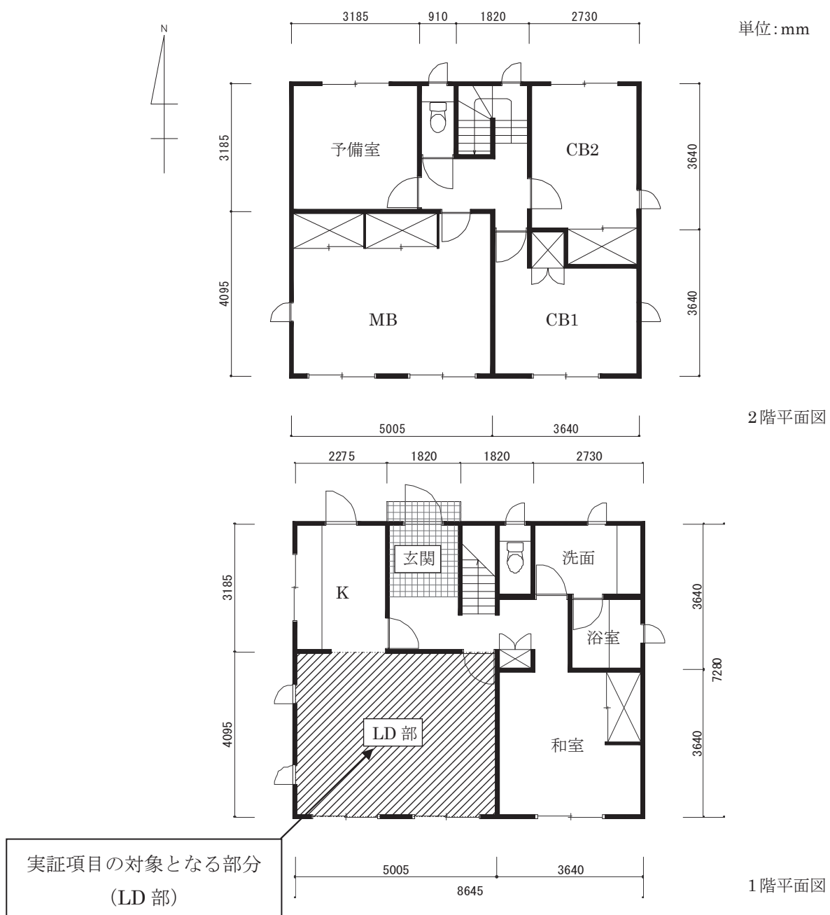
図 4-1 計算用住宅モデル（平面図）
